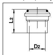
Втулки под пайку
