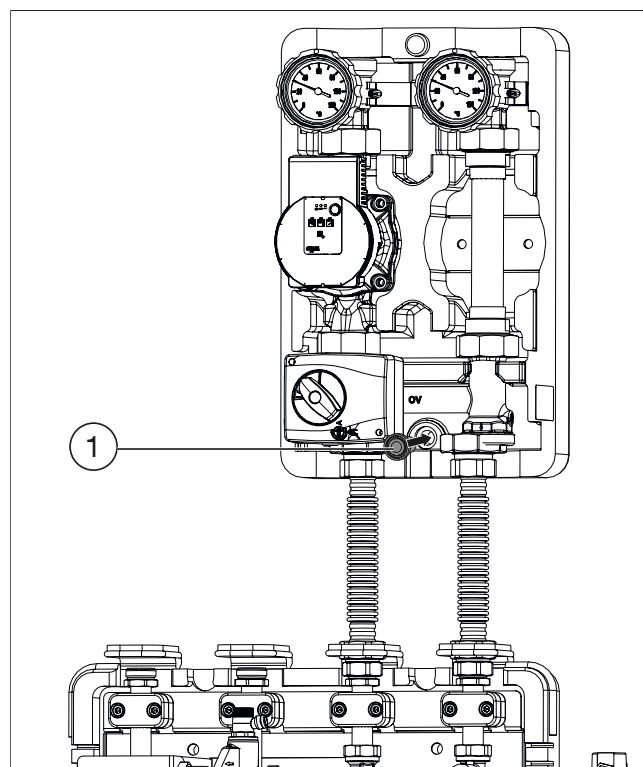
Abb. 39: Distanzstück Regumat M3 einsetzen
