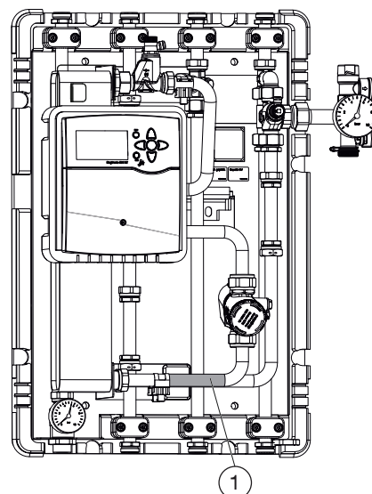
Abb. 42: Hausübergabestation erden
