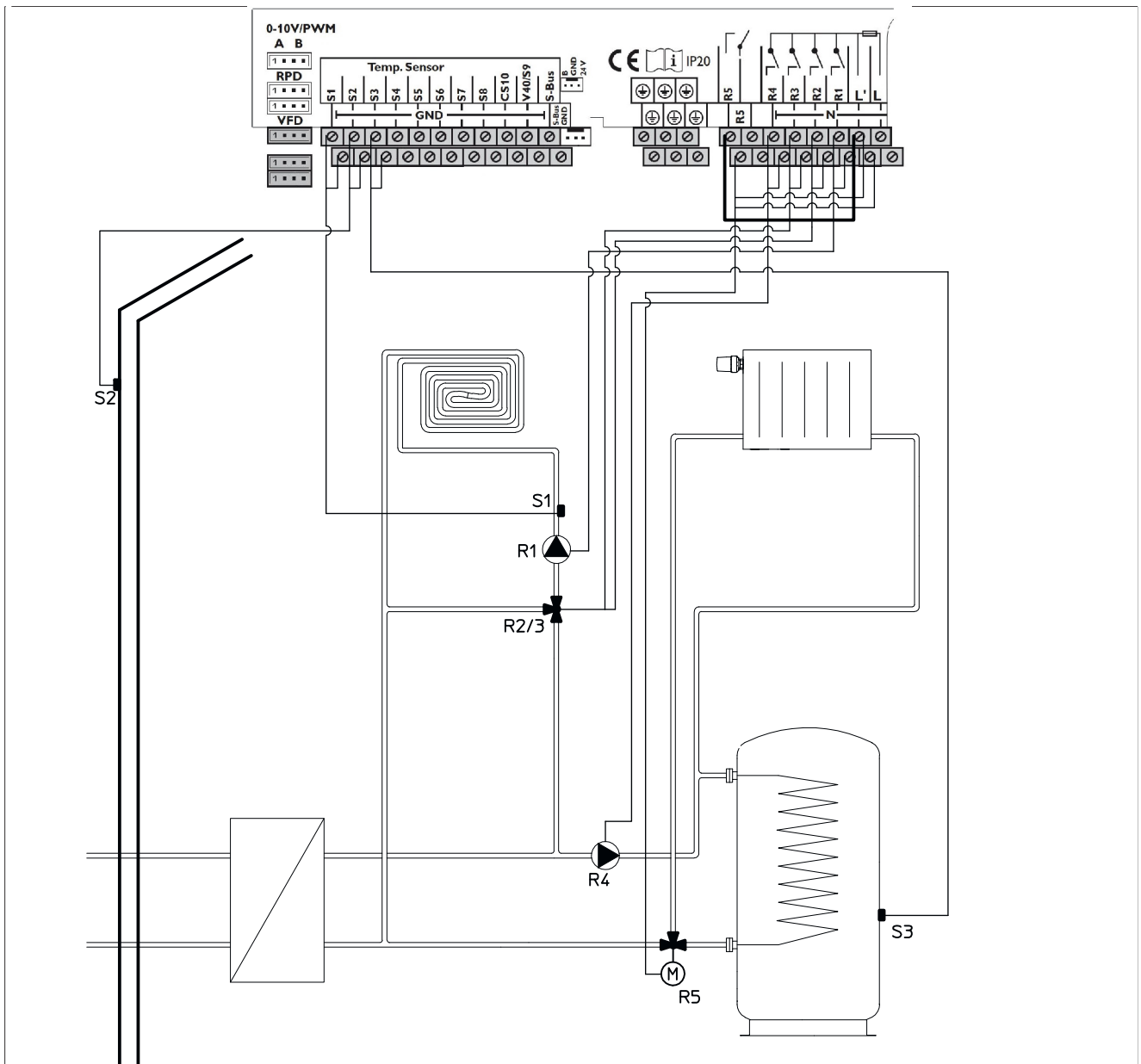
Abb. 57: Schema 10, ein gemischter und ein ungemischter Heizkreis, indirekte Trinkwasserwärmung
