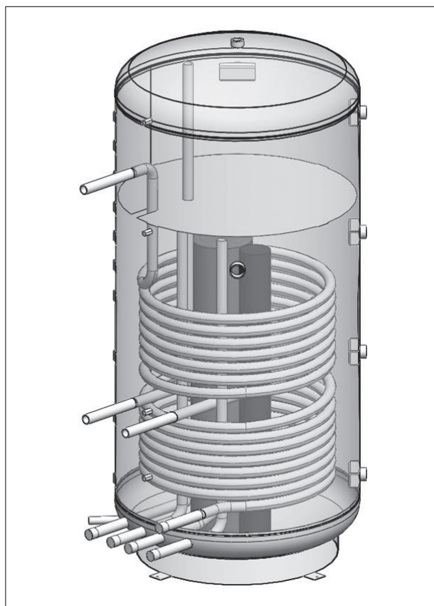
Solarer Pufferspeicher
