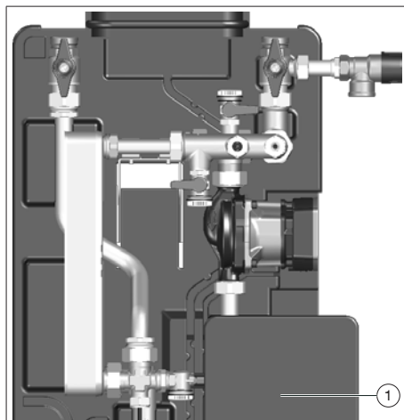
Fig. 4: Ouverture du régulateur
