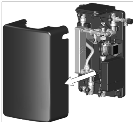
Fig. 1: Retrait de la coquille supérieure
