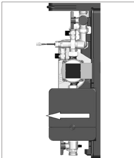
Fig. 2: Retrait du régulateur
