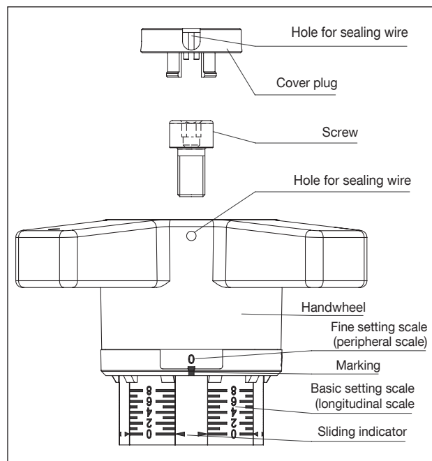
Dimensions
