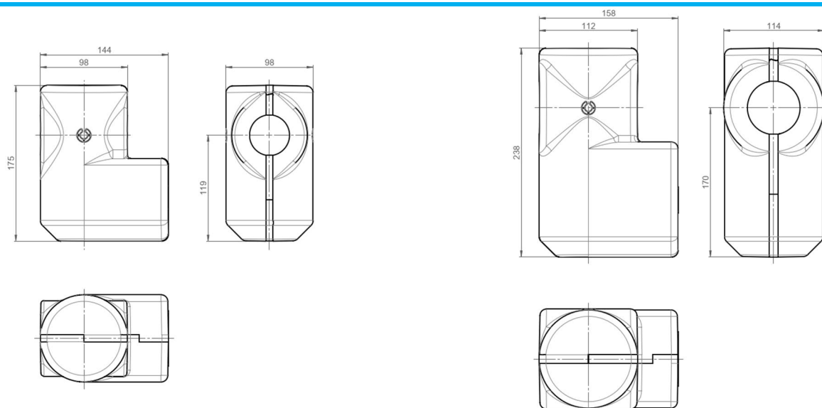
Pour DN 20 et DN 25, montage horizontal (réf. 1124091)
