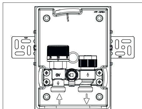
Fig. 7 : « Unibox T-RTL vario » avec équerres
