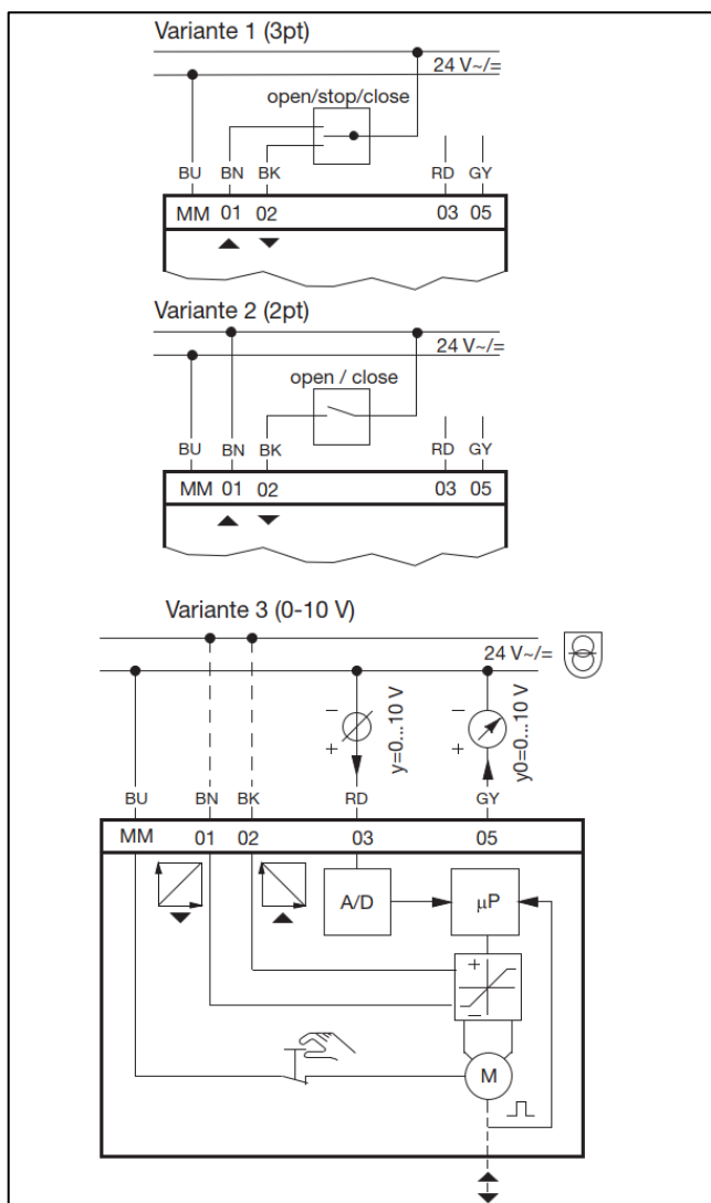
Schaltpläne Art.-Nr.: 1158011
