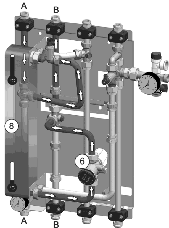
Abb. 3: Primärseite Übergabestation (Beispiel Anschluss von oben)
