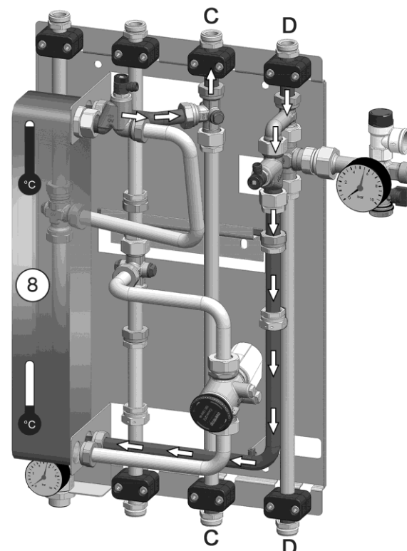
Abb. 4 Sekundärseite Übergabestation (Beispiel Anschluss von oben)
