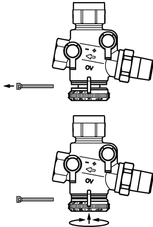
Abb. 26: Einstellung des max. Volumenstroms am „Cocon QTZ“
