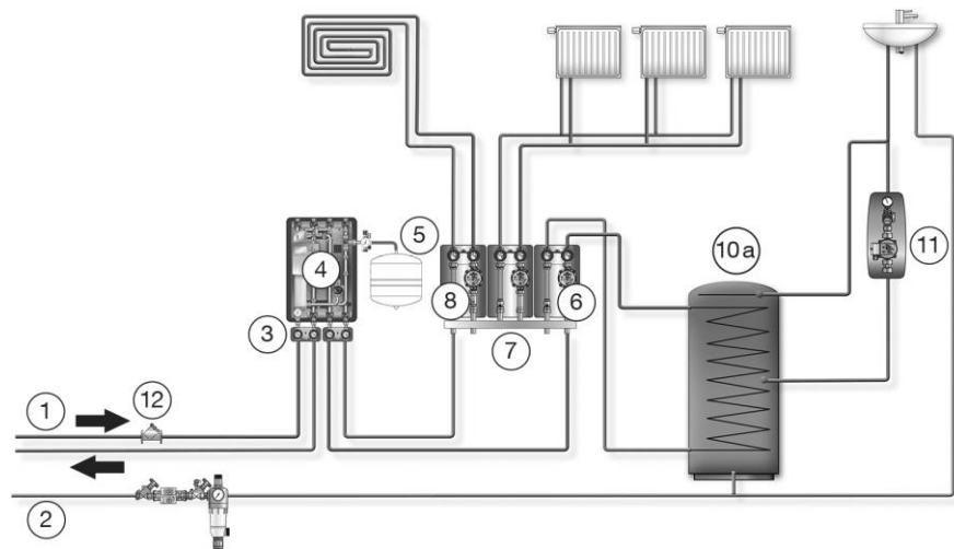
Abb. 6: Installation mit ungemischtem und gemischtem Heizkreis sowie indirekter Trinkwassererwärmung
