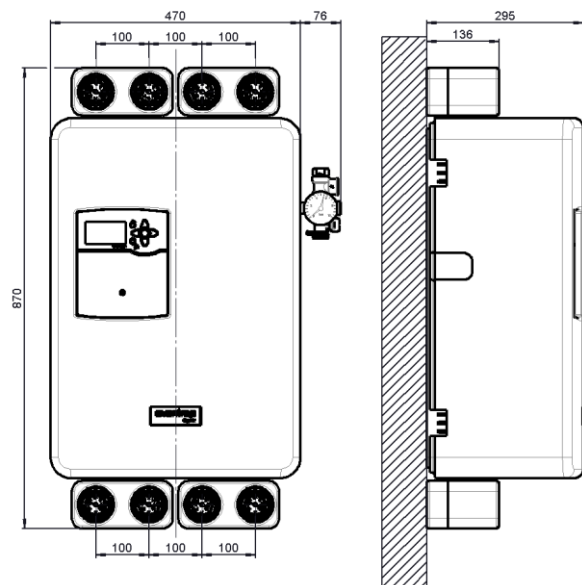
Abb. 9: „Regudis H-HT“ mit Kugelhahnanschluss Sets
