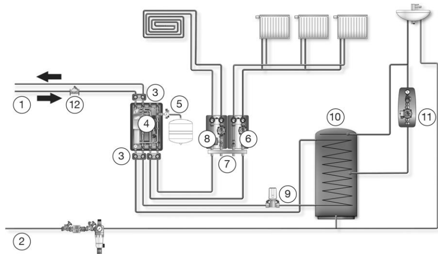
Abb. 5: Installation mit ungemischtem und gemischtem Heizkreis sowie direkter Trinkwassererwärmung
