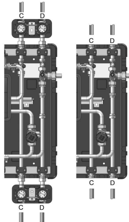
Abb. 19: Sekundärseitiger Anschluss von bis zu zwei Heizkreisen (Vorlauf = C; Rücklauf = D) an der Station.
