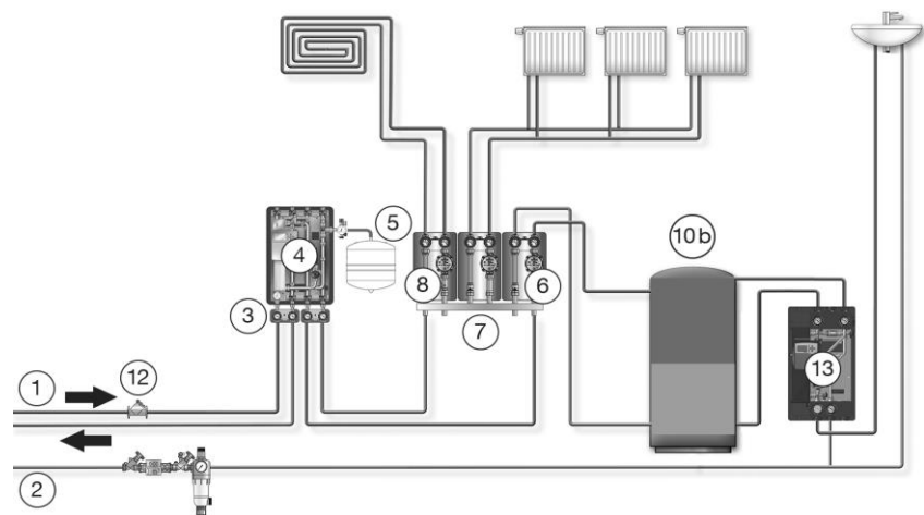
Abb. 7: Installation mit ungemischtem und gemischtem Heizkreis sowie indirekter Pufferspeicherbeladung zur Trinkwassererwärmung im Durchflussprinzip
