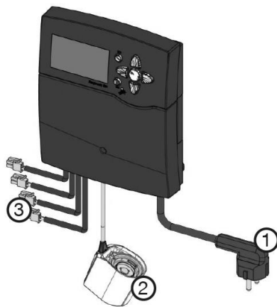
Abb. 1: Regler mit Anschlüssen.
