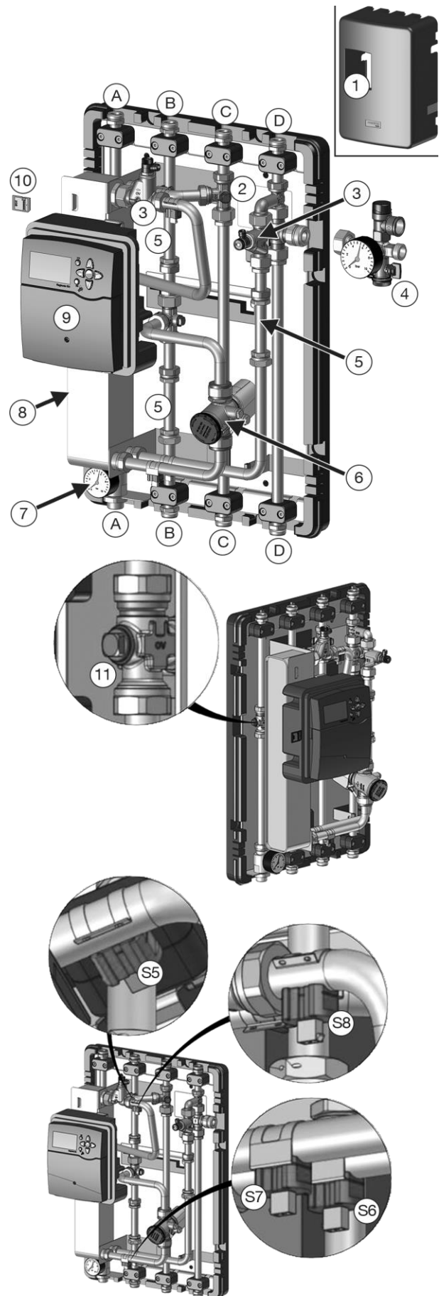
Abb. 2: Übersicht Übergabestation „Regudis H-HT“
