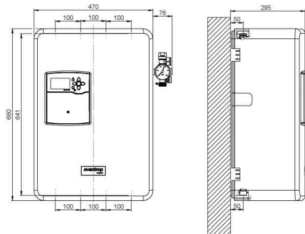
Abb. 8: Abmessungen „Regudis H-HT“
