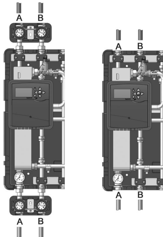
Abb. 17: Primärseitiger Anschluss der Versorgungsleitungen (Vorlauf = A; Rücklauf = B) entweder von oben oder von unten.
