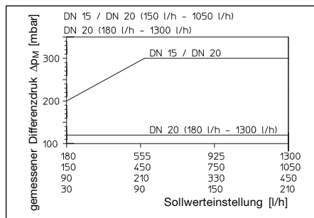
Abb. 5.1 Differenzdruck / SollwertEinstellung
