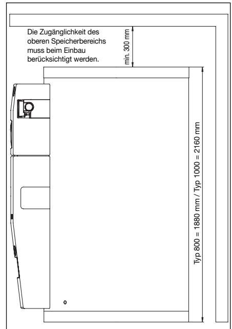
Abb. 4 Einbaumaße
