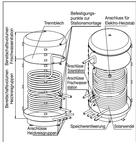
Abb. 43 Funktionsschnitt
