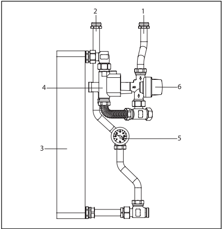
Fig. 32 Circuit secondaire
