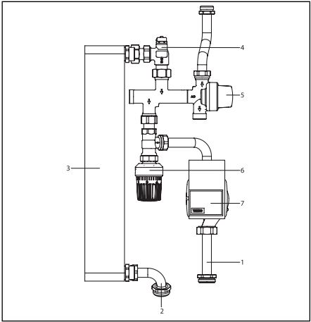
Fig. 31 Circuit primaire
