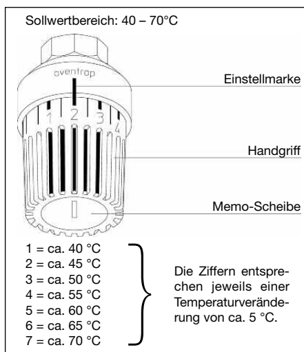
Abb. 34 Temperaturregler
