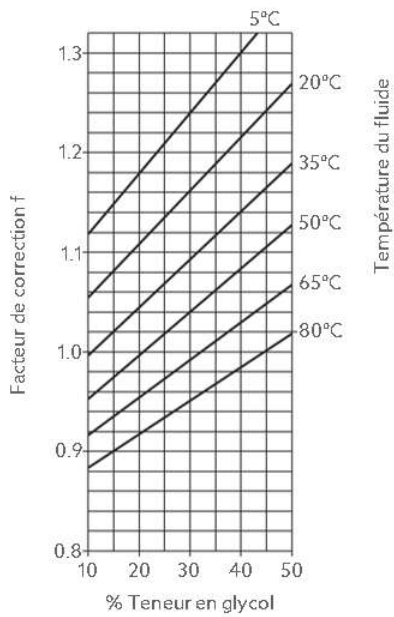
Facteur de correction f pour l'éthylène glycol
