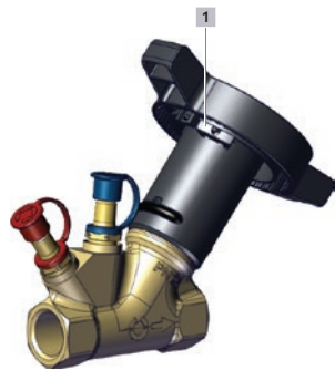
Fig. 3: Posición de la pinza delimitadora
