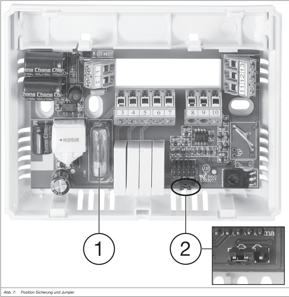
Abb. 7: Position Sicherung und Jumper
