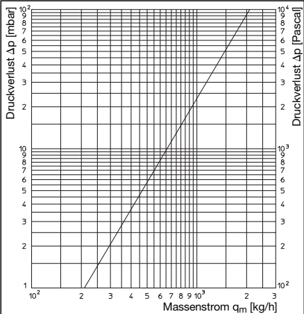
Diagramm 1: Druckverlust Wärmemengenzähler Anschluss-Set 1, DN 20
