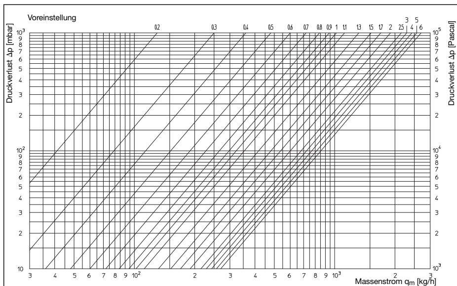
Diagramm 2: Druckverlust „Hycococon VTZ“ Strangreguliventil DN 20
