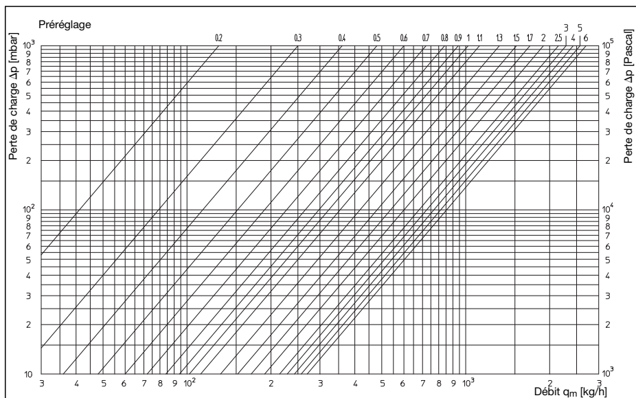
Diagramme 2: Perte de charge robinet d'équilibrage «Hycococon VTZ» DN 20
