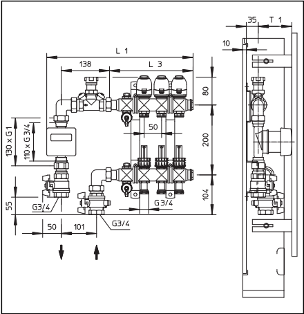
Illustr. 1: Exemple: Jeu de raccordement no. 1 pour compteurs de calories, modèle équerre, et distributeur/collecteur en acier inoxydable «Multidis SF» pour installations de surfaces chauffantes, longueurs et profondeur
