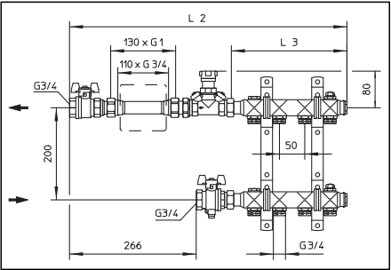
Abb. 2: Wärmemengenzähler-Anschluss-Set 1, Durchgangsform, und „Multidis SH“ Edelstahl-Verteiler für Heizkörperanbindung, Baulängen
