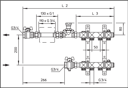
Illustr. 2: Exemple: Jeu de raccordement no. 1 pour compteurs de calories, modèle droit, et distributeur/collecteur en acier inoxydable «Multidis SH» pour le raccordement de radiateurs, longueurs et profondeur
