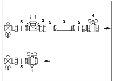
Abb. 4: Wärmemengenzähler-Anschluss-Set 1, Durchgangsform, Lieferumfang und Anordnung der Komponenten bei Rechtsanschluss
