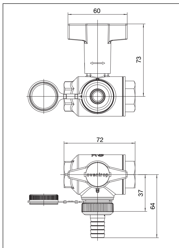
Dimensiuni
