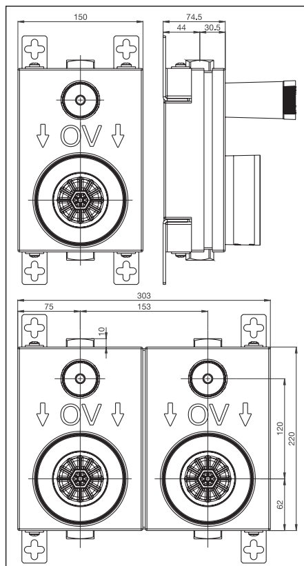
Fig. 4.1 Dimensions et cotes de raccordement
