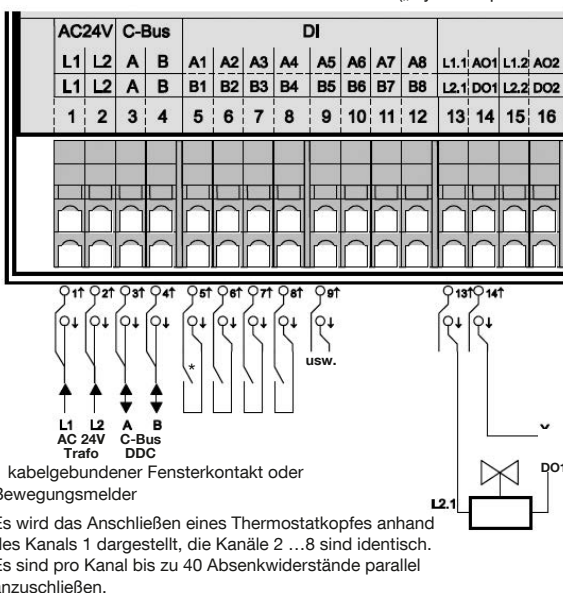
Anschlussbeispiele DynaTemp CR-BX „RM-C F8“
