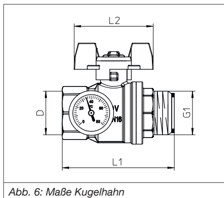
Abb. 6: Maße Kugelhahn
