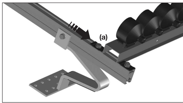
Fig. 13: Déplacer la plaque de serrage (a) vers le «bas». Visser à fond les deux vis M8.
