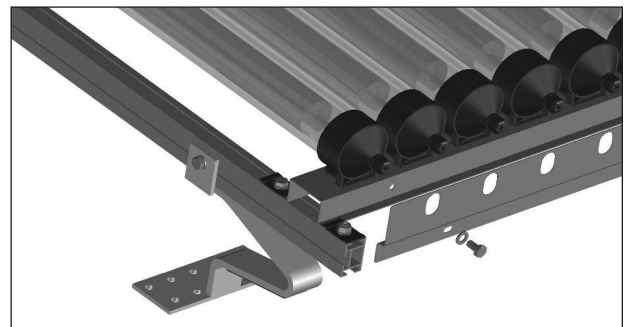
Abb. 25: Winkelblech an der Unterseite der Fußschiene montieren
