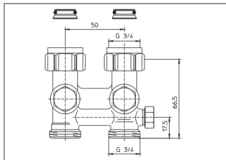
Fig. 3 Modèle droit, G ¾ écrou x G ¾ mâle
