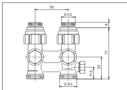
Fig. 4 Modèle droit, G ½ mâle x G ¾ mâle
