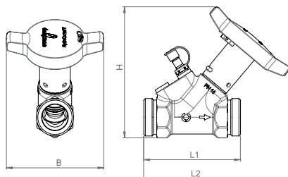
Abb. 3: Encombremes vue de côté - Version avec filetage mâle
