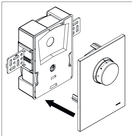
Fig. 11: Pose du capot avec poignée manuelle
