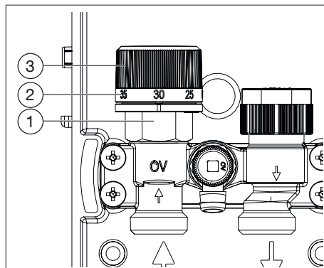
Abb. 4: Handrad
