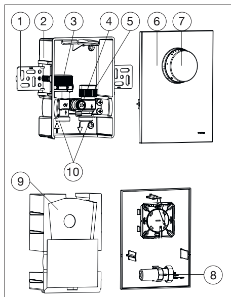
Fig. 2: Configuration de l'« Unibox T RTL »
