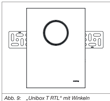
Abb. 9: „Unibox T RTL“ mit Winkeln
