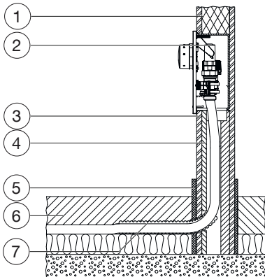
Abb. 7: Einbauquerschnitt
