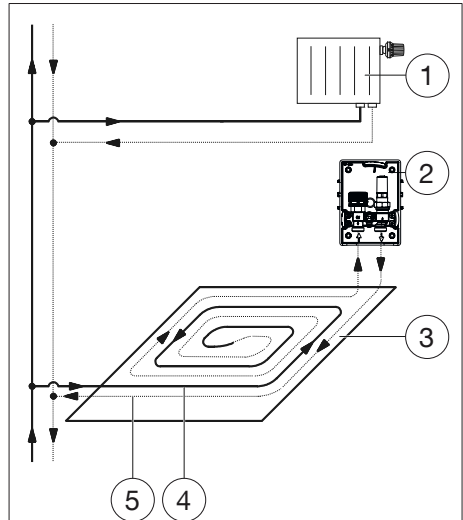
Abb. 8: Anschluss
