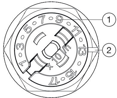
Abb. 5: Einstellung Ventileinsatz „QM“
