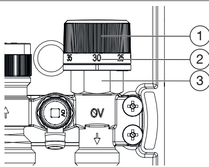
Abb. 4: Handrad
