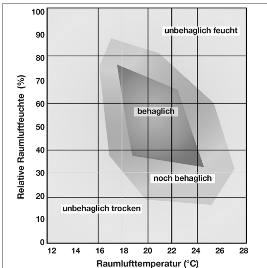
Abb. 59: „Behaglichkeitsdiagramm“
