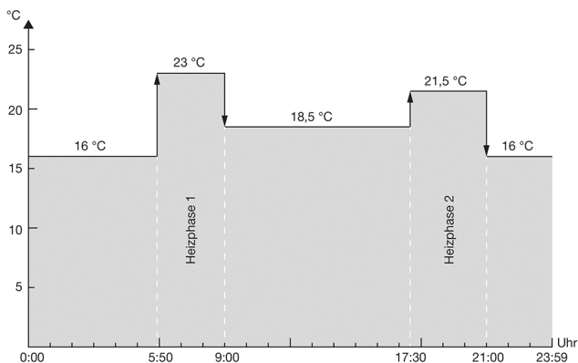
Abb. 38: Die im Beispiel programmierten Heiz-/Absenkenphasen in 24-Stunden-Ansicht:
