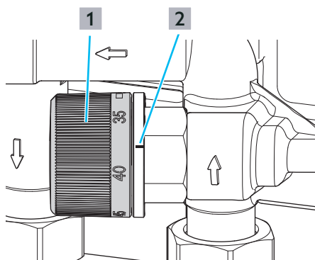
Abb. 33: Temperaturvorhalte-Regelset einstellen
