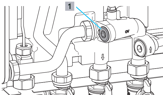
Abb. 42: Filtereinsatz reinigen
