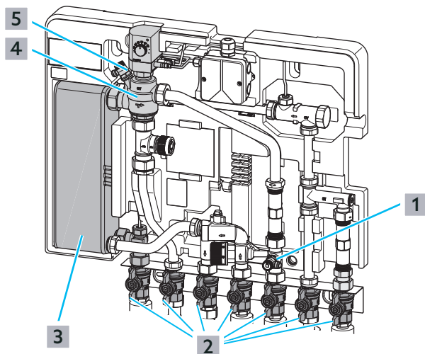
Abb. 36: Wärmeübertrager ausbauen und reinigen
