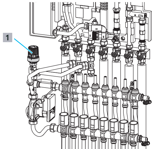
Abb. 34: Heizkreistemperatur einstellen
