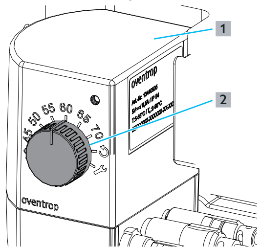
Abb. 32: Warmwassertemperatur einstellen
