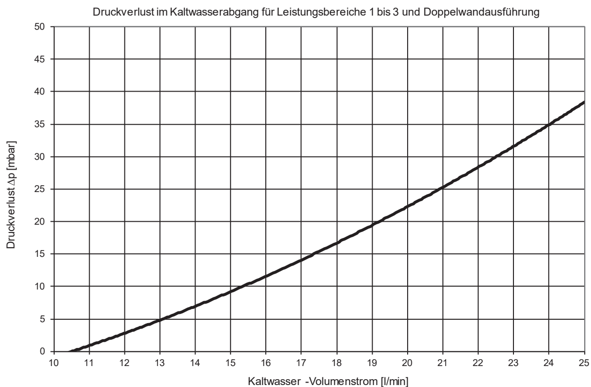
Abb. 50: Druckverlust im Kaltwasserabgang
