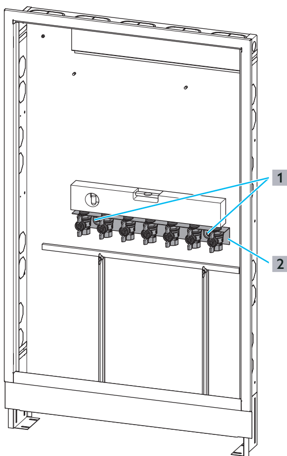
Abb. 13: Kugelhahn-Anschlusset montieren
