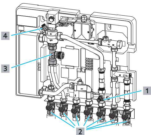
Abb. 31: Kugelhähne und Ventile einstellen
