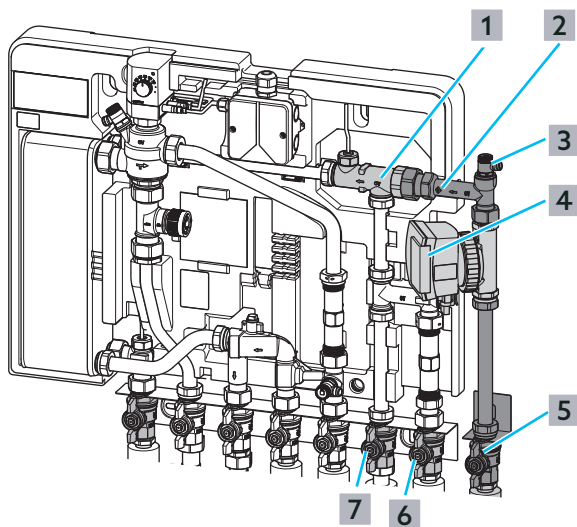
Abb. 22: Trinkwasser-Zirkulationsmodul montieren
