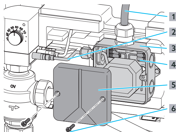
Abb. 27: Station elektrisch anschließen
