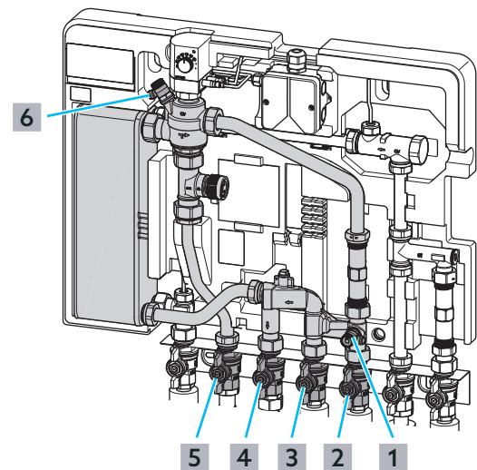
Abb. 28: Heizkreis füllen und entlüften
