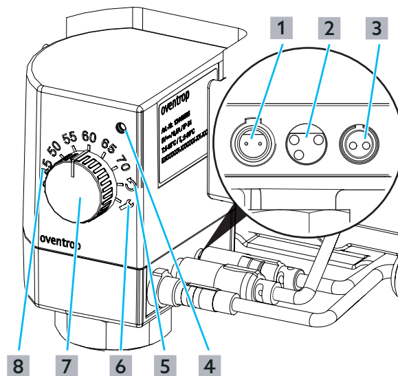
Abb. 7: Stellantrieb mit integrierter Trinkwassertemperaturregelung
