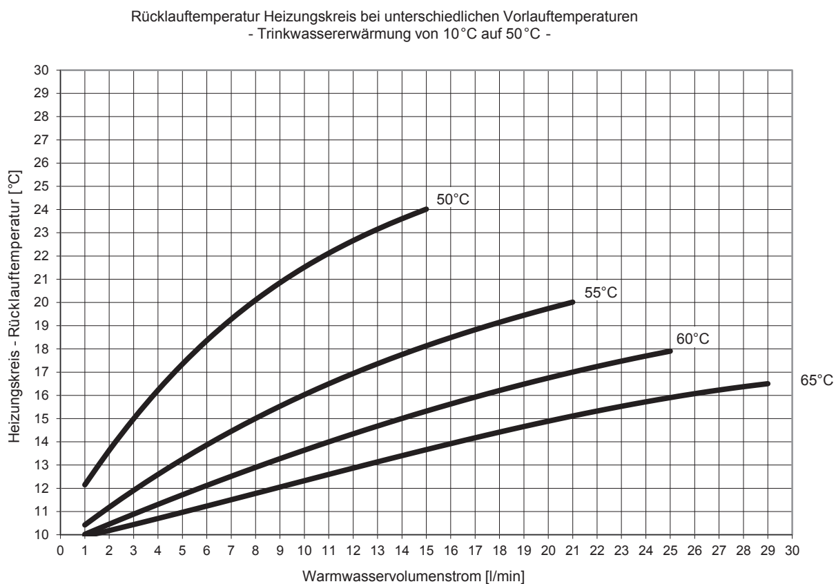
Abb. 62: Leistungsbereich 2, Trinkwassererwärmung auf 50 °C
