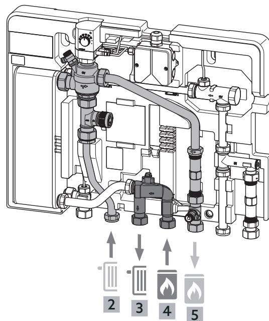
Abb. 4: Heizbetrieb
