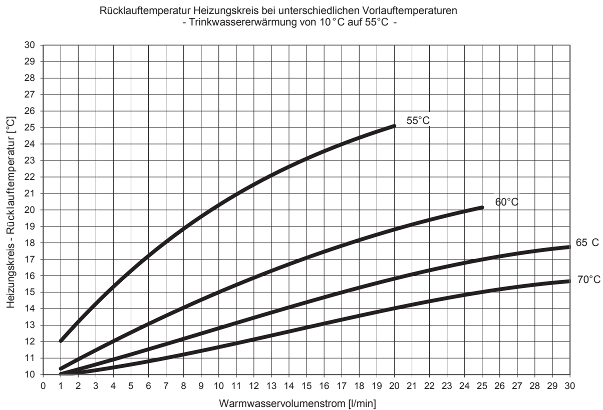
Abb. 72: Leistungsbereich 3, Trinkwassererwärmung auf 55 °C
