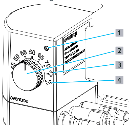
Abb. 35: Statusmeldungen und Fehlermeldungen am Stellantrieb
