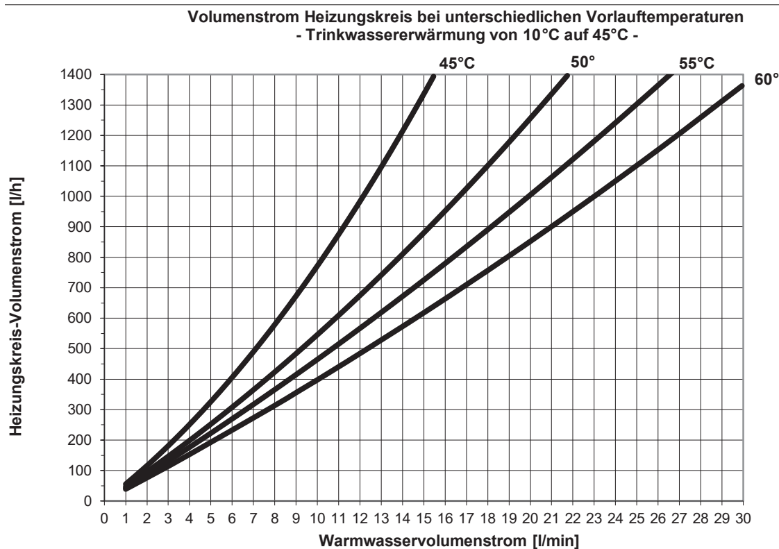
Abb. 75: Doppelwandausführung, Trinkwassererwärmung auf 45 °C
