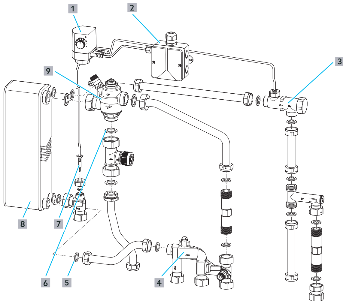
Abb. 11: Ersatzteile
