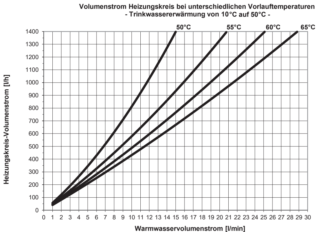
Abb. 77: Doppelwandausführung, Trinkwassererwärmung auf 50 °C
