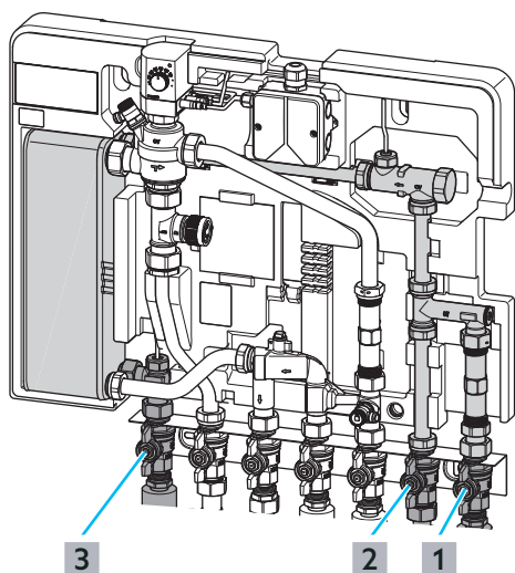
Abb. 29: Trinkwasserkreis füllen
