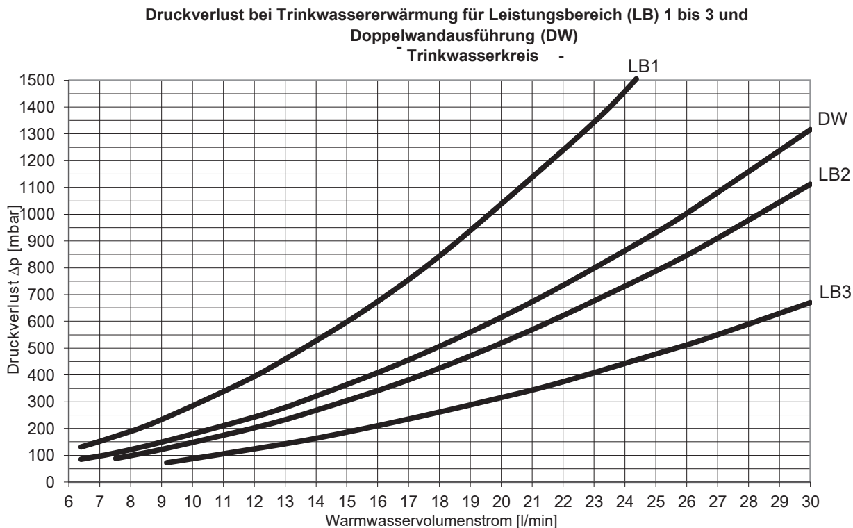
Abb. 47: Druckverlust im Trinkwasserkreis
