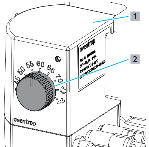
Abb. 45: Warmwassertemperatur einstellen
