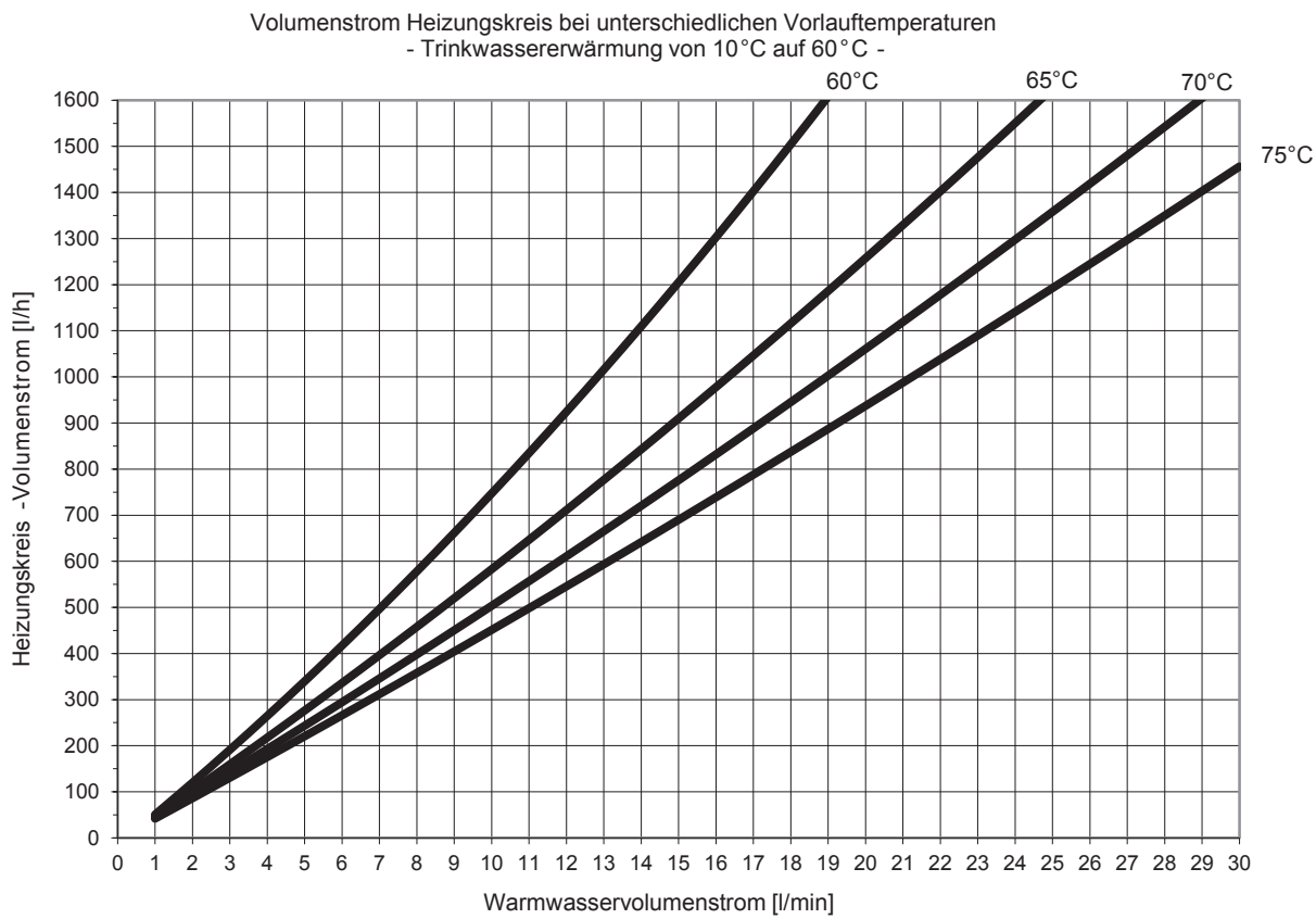
Abb. 73: Leistungsbereich 3, Trinkwassererwärmung auf 60 °C
