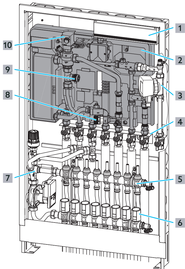
Abb. 6: Systembeispiel mit Einbauschrank, Trinkwasser-Zirkulation und Flächenheizung
