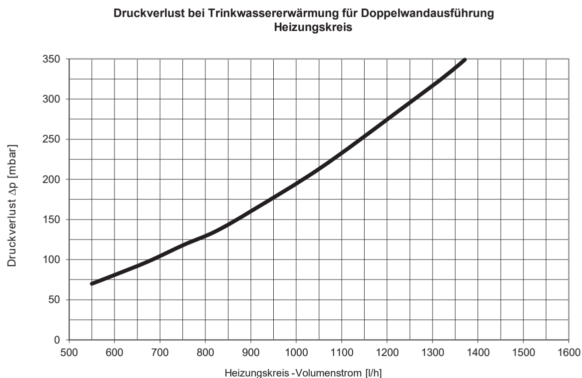
Abb. 49: Druckverlust im Heizungskreis Doppelwandausführung
