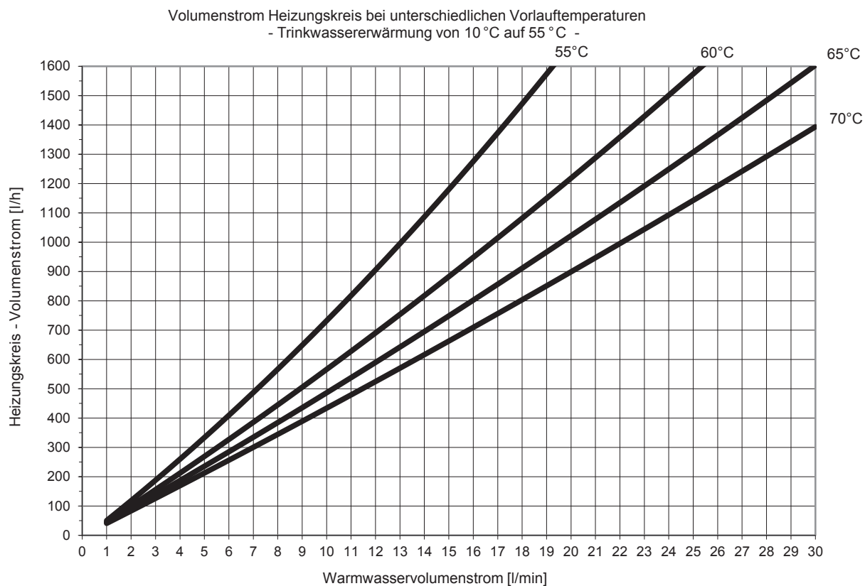
Abb. 71: Leistungsbereich 3, Trinkwassererwärmung auf 55 °C
