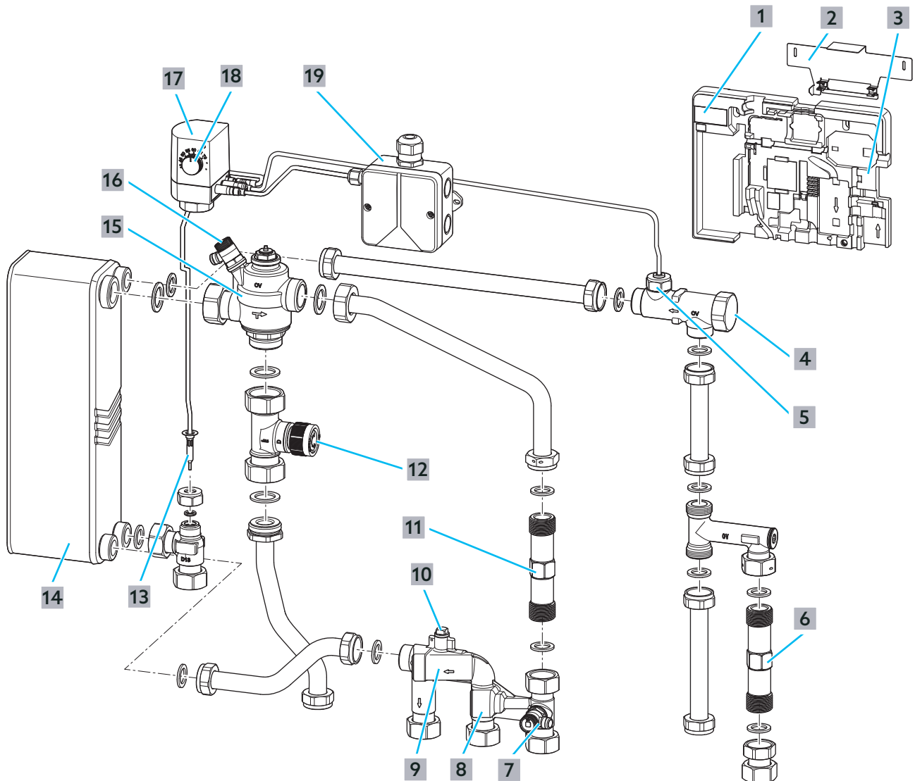
Abb. 3: Übersicht Wohnungsstation Regudis W-HTE
