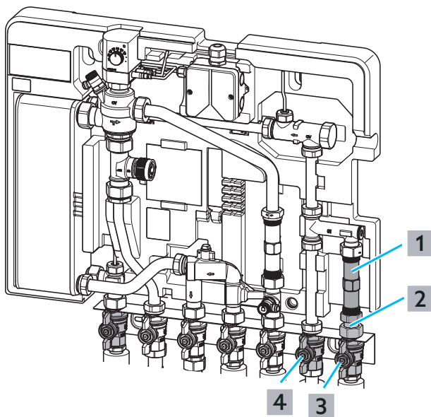
Abb. 21: Wasserzähler montieren
