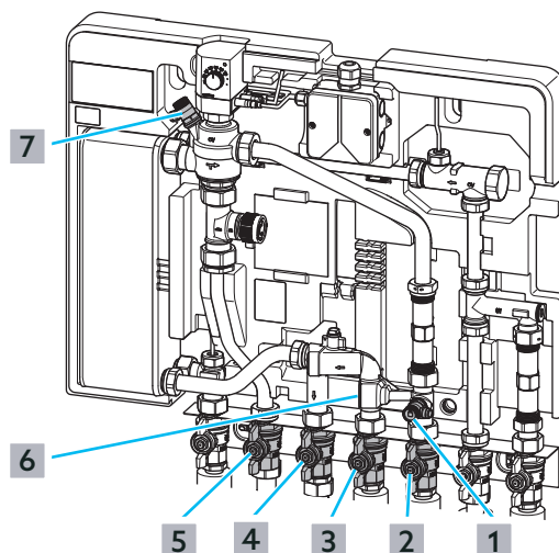
Abb. 23: Station entleeren (Heizungskreis)
