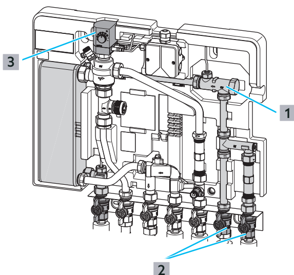
Abb. 37: Volumenstromsensor prüfen und reinigen
