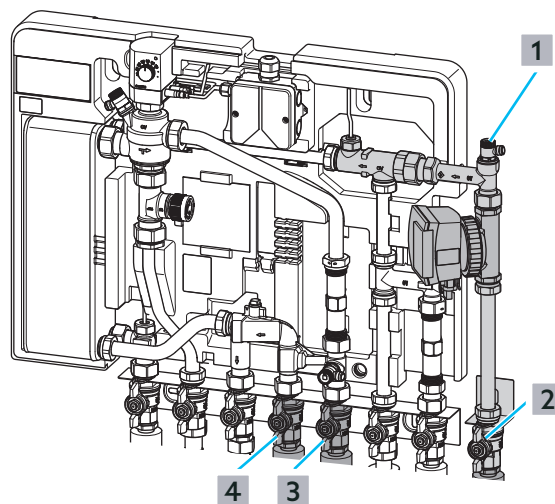
Abb. 30: Zirkulationsleitung
