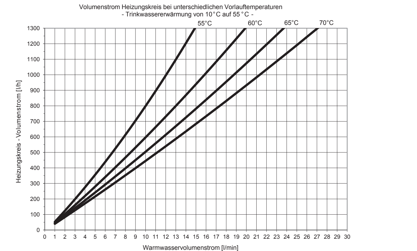
Abb. 63: Leistungsbereich 2, Trinkwassererwärmung auf 55 °C
