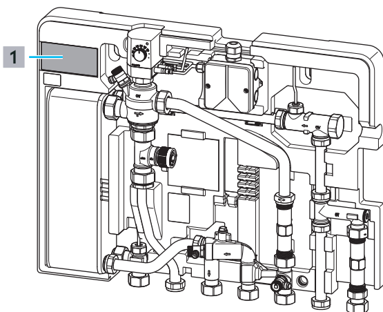
Abb. 1: Position des Typenschilds
