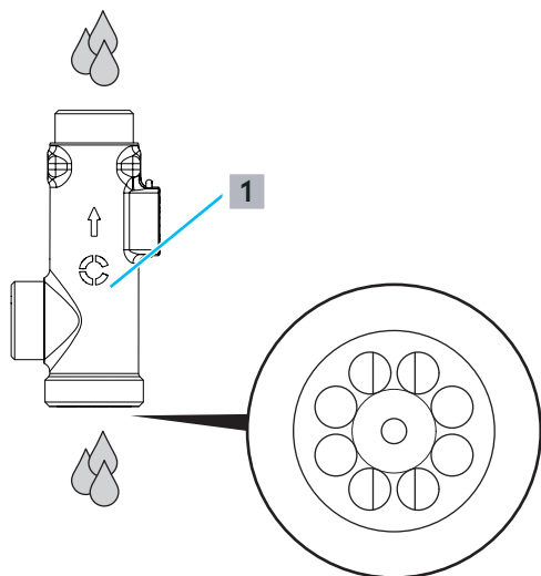
Abb. 40: Volumenstromsensor unter fließendem Wasser reinigen
