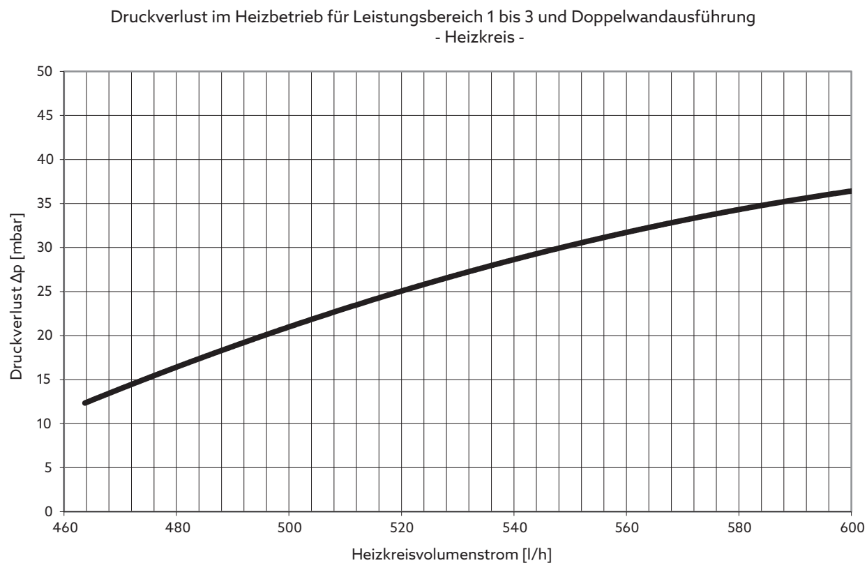
Abb. 46: Druckverlust im Heizbetrieb
