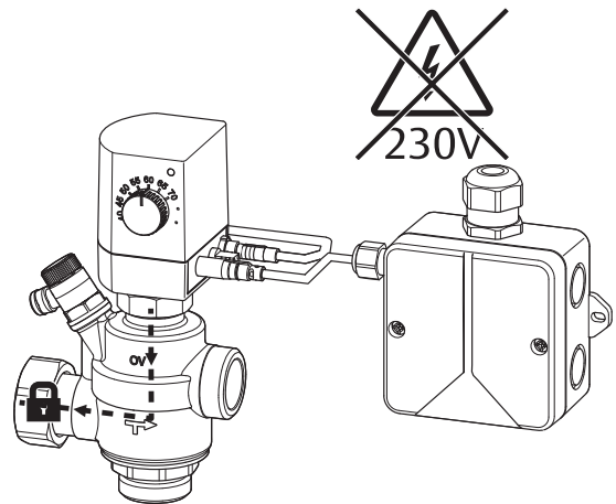
Abb. 2: Regelventil schließt bei Stromausfall
