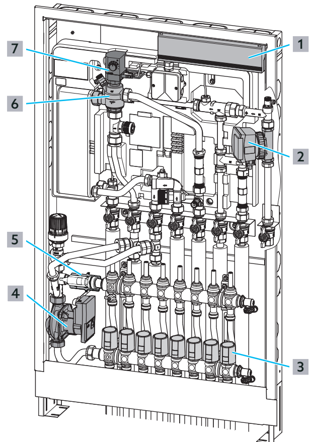
Abb. 44: Elektrische Komponenten prüfen
