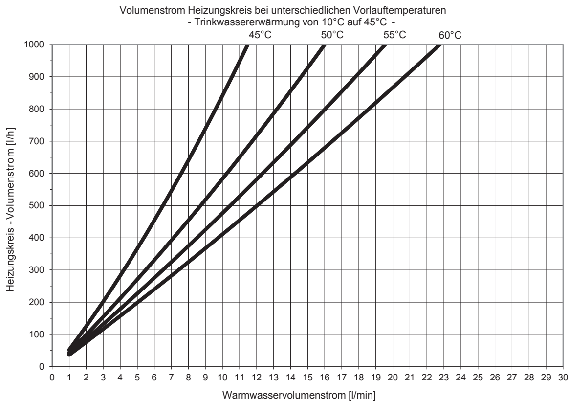
Abb. 51: Leistungsbereich 1, Trinkwassererwärmung auf 45 °C
