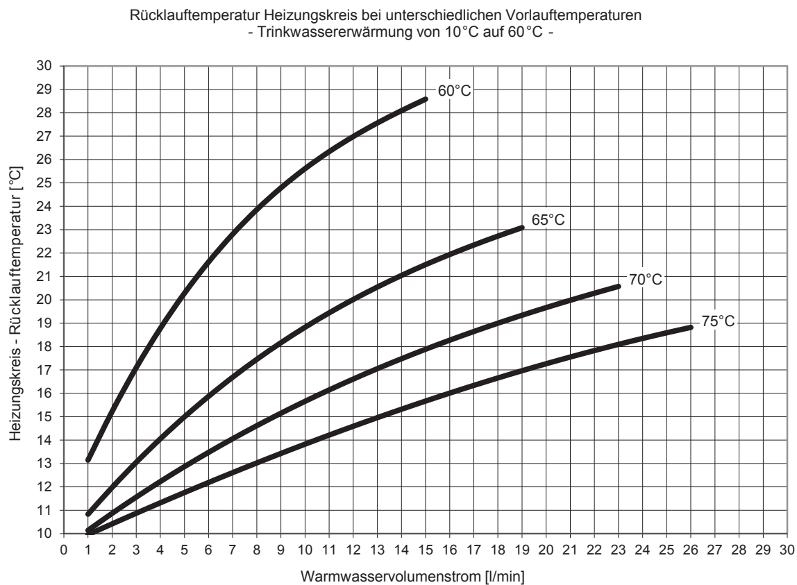
Abb. 66: Leistungsbereich 2, Trinkwassererwärmung auf 60 °C
