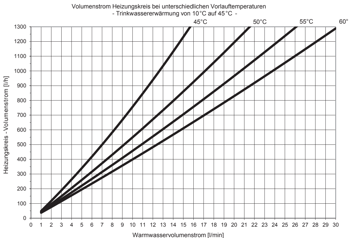
Abb. 59: Leistungsbereich 2, Trinkwassererwärmung auf 45 °C
