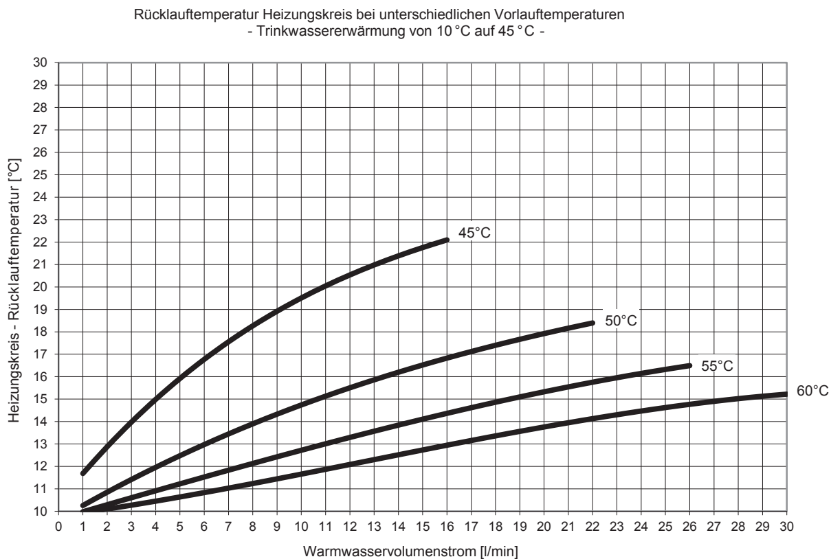
Abb. 60: Leistungsbereich 2, Trinkwassererwärmung auf 45 °C
