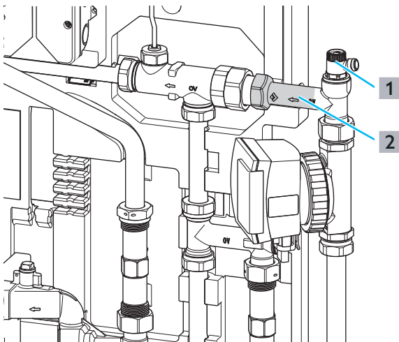
Abb. 43: Sperrventil prüfen
