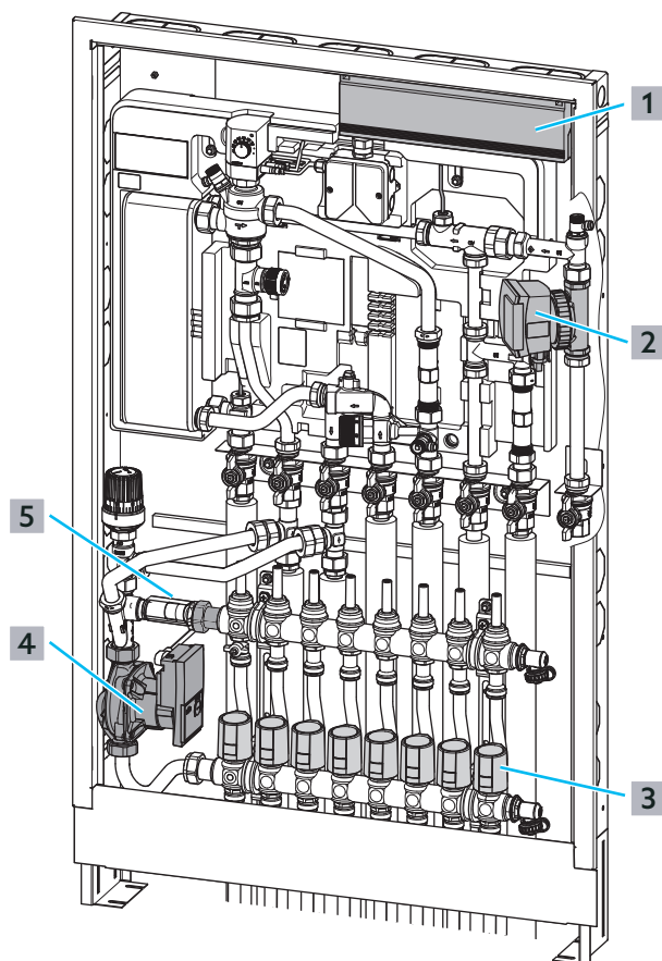
Abb. 26: Stellantriebe und Pumpe für Flächenheizung elektrisch anschließen
