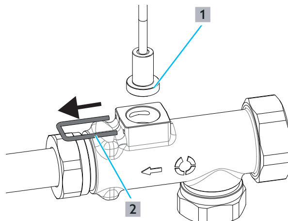
Abb. 38: Sicherungsklammer lösen
