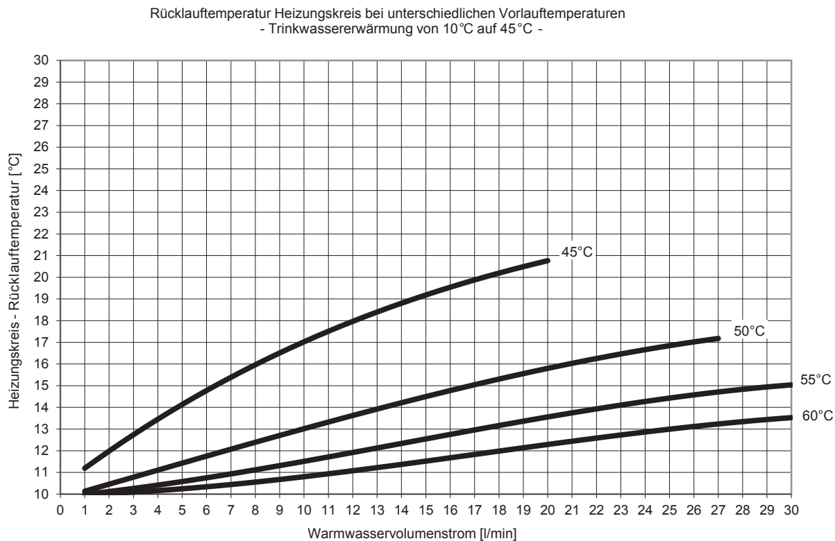
Abb. 68: Leistungsbereich 3, Trinkwassererwärmung auf 45 °C
