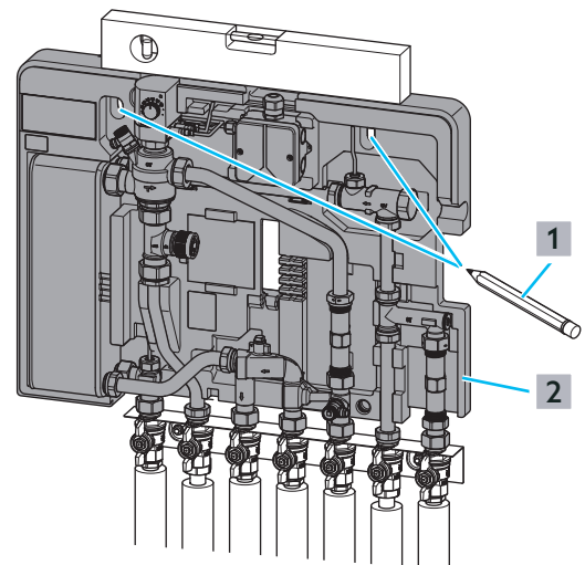
Abb. 17: Station ausrichten und anzeichnen
