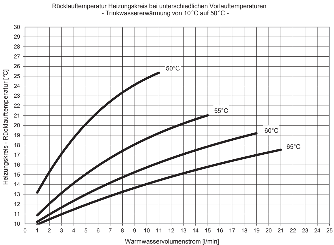
Abb. 54: Leistungsbereich 1, Trinkwassererwärmung auf 50 °C
