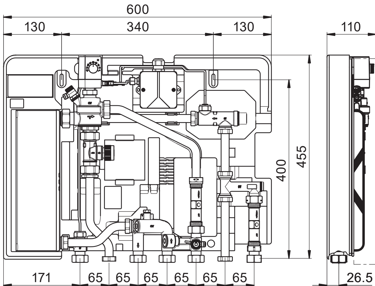
Abb. 9: Abmessungen
