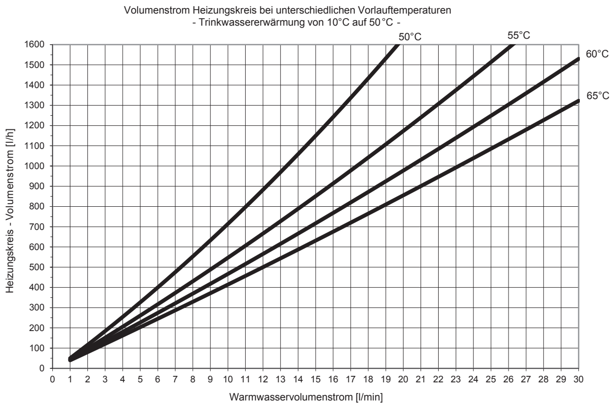
Abb. 69: Leistungsbereich 3, Trinkwassererwärmung auf 50 °C
