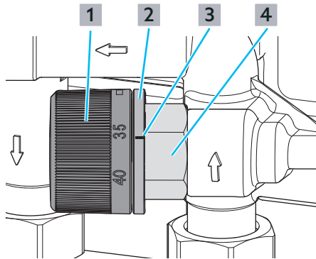
Abb. 24: Temperaturvorhalte-Regelset montieren
