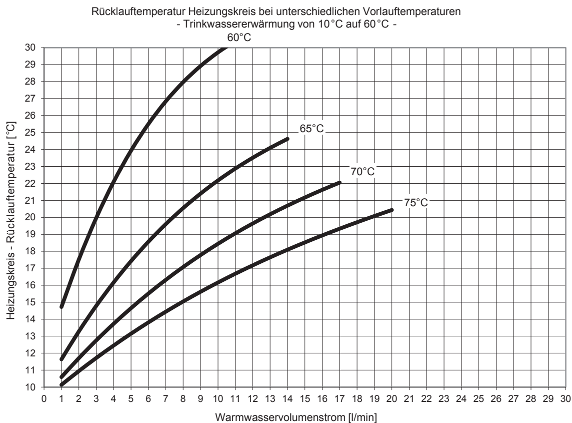
Abb. 58: Leistungsbereich 1, Trinkwassererwärmung auf 60 °C
