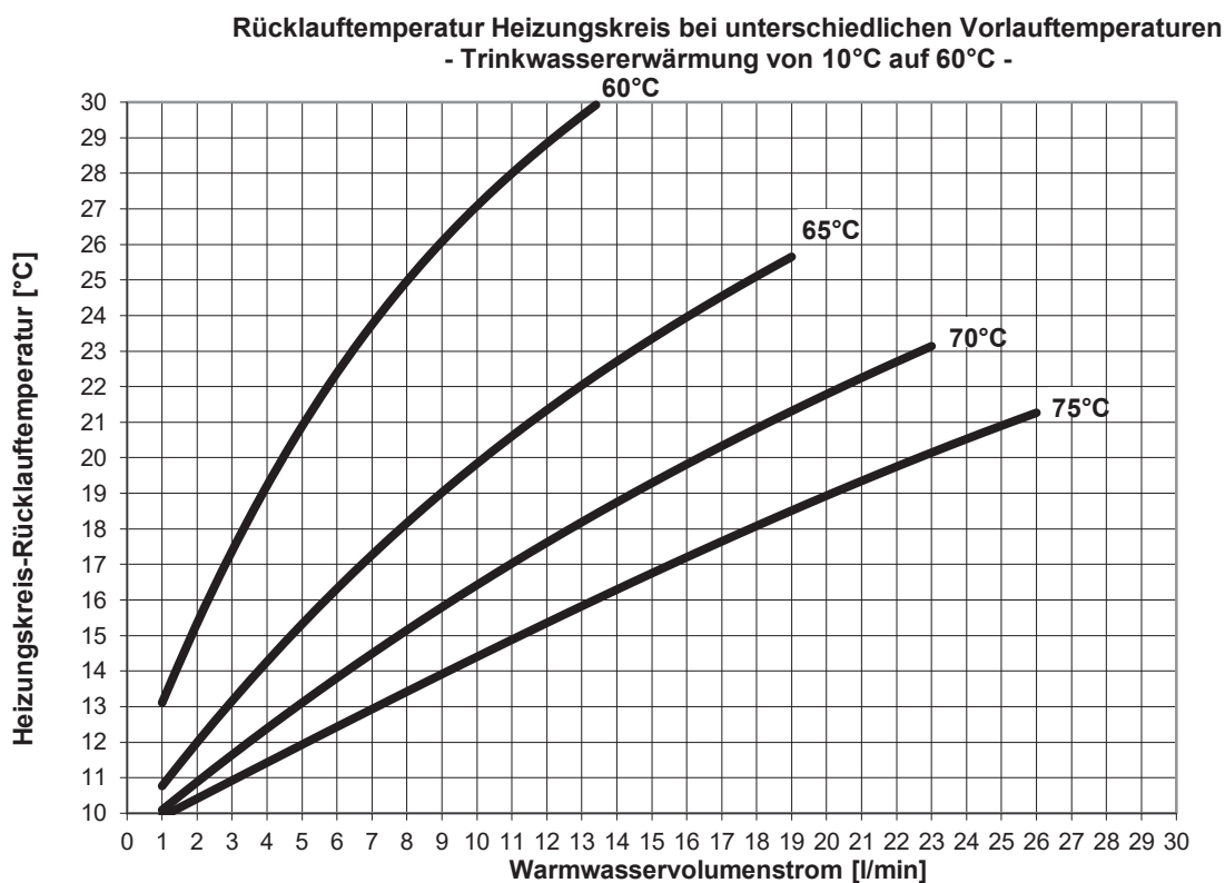
Abb. 82: Doppelwandausführung, Trinkwassererwärmung auf 60 °C
