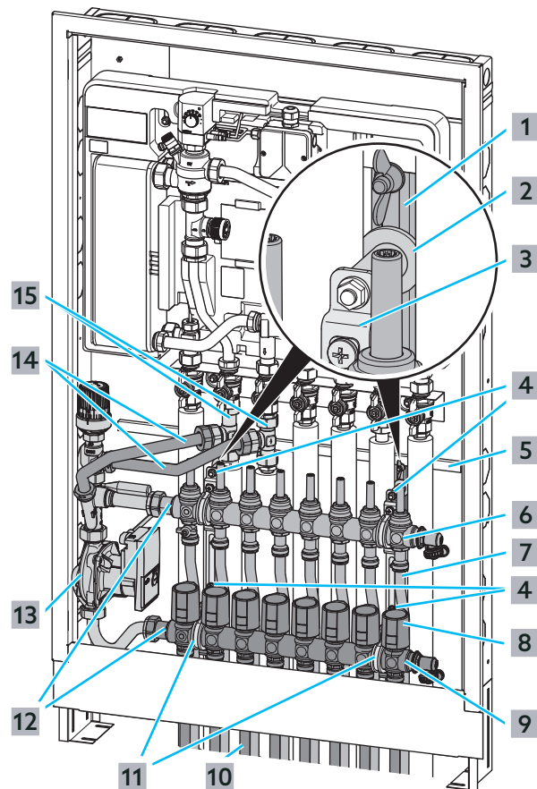
Abb. 15: Vorlauftemperatur-Regelmodul montieren
