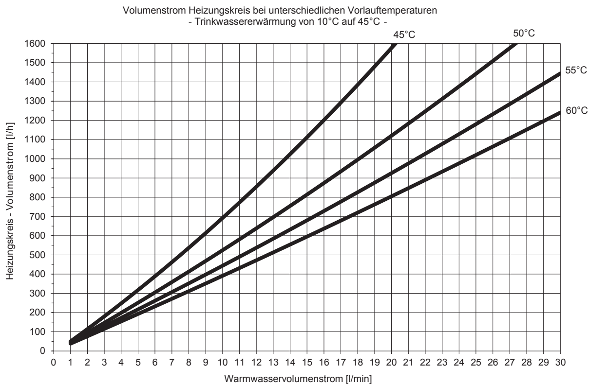
Abb. 67: Leistungsbereich 3, Trinkwassererwärmung auf 45 °C
