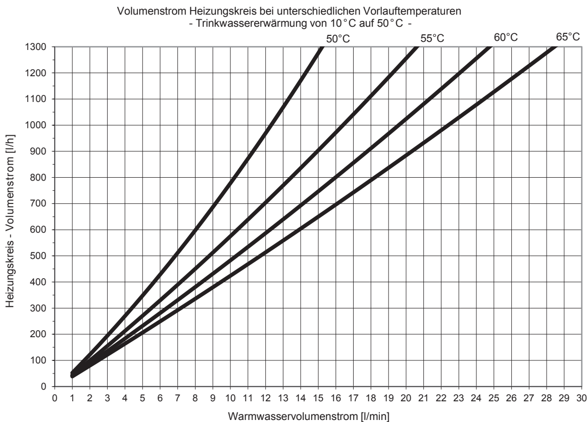
Abb. 61: Leistungsbereich 2, Trinkwassererwärmung auf 50 °C
