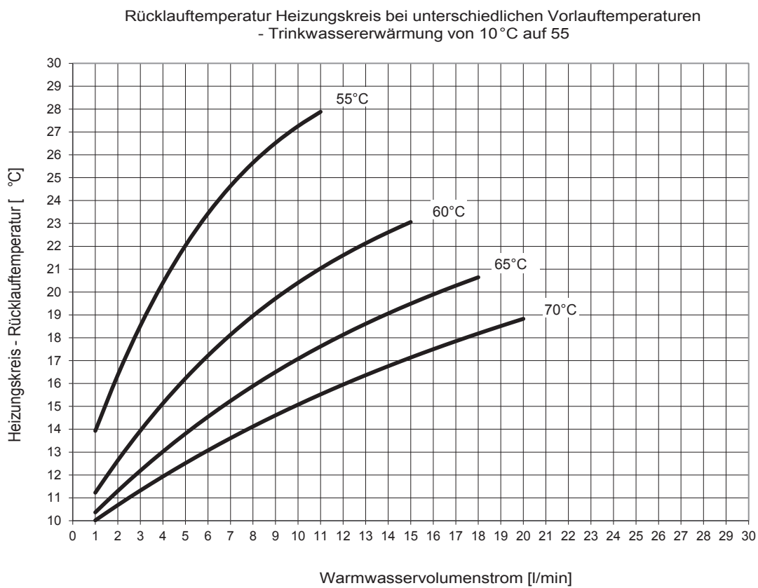
Abb. 55: Leistungsbereich 1, Trinkwassererwärmung auf 55 °C
