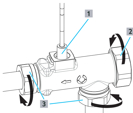
Abb. 41: Volumenstromsensor einbauen
