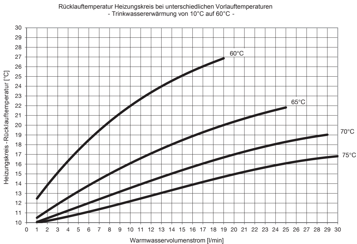
Abb. 74: Leistungsbereich 3, Trinkwassererwärmung auf 60 °C
