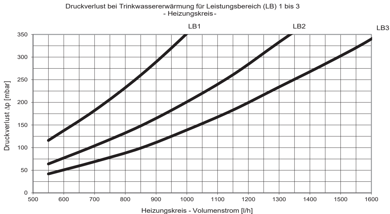
Abb. 48: Druckverlust im Heizungskreis Leistungsbereich 1-3
