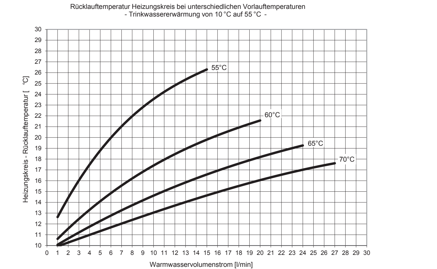
Abb. 64: Leistungsbereich 2, Trinkwassererwärmung auf 55 °C
