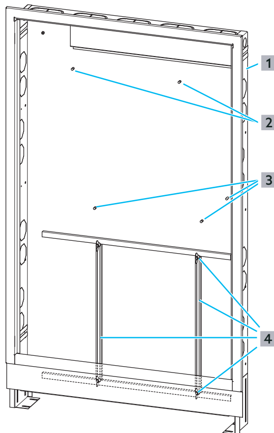
Abb. 12: Oventrop Einbauschränk vorbereiten
