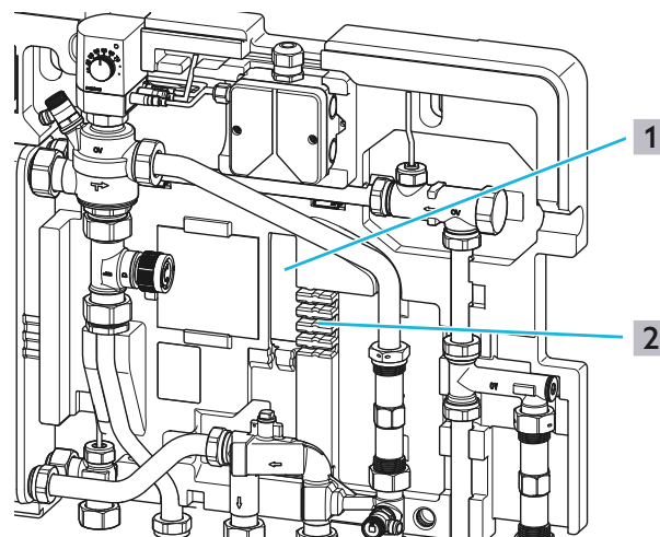
Abb. 20: Aussparung und Kabelführungen in der Unterschale
