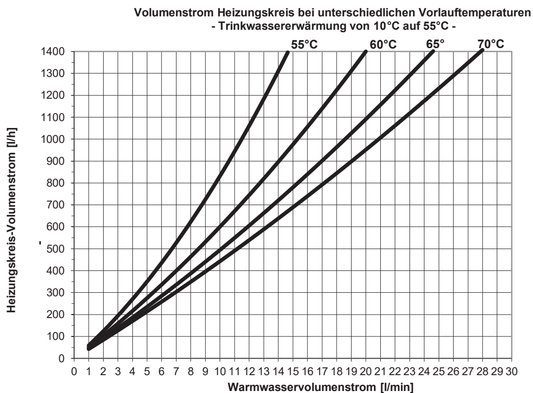
Abb. 79: Doppelwandausführung, Trinkwassererwärmung auf 55 °C
