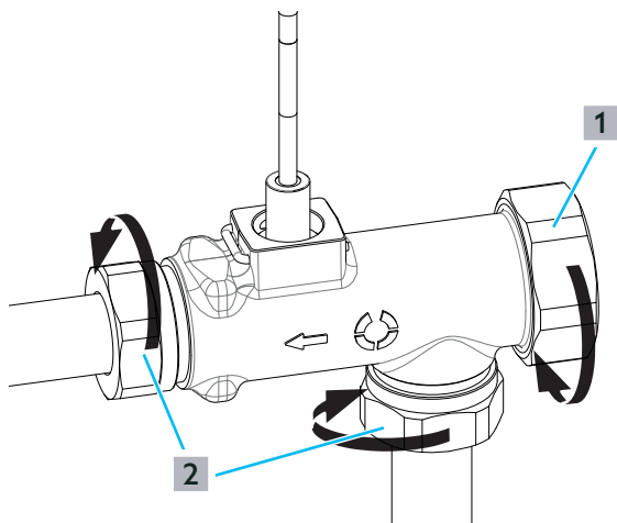
Abb. 39: Volumenstromsensor ausbauen
