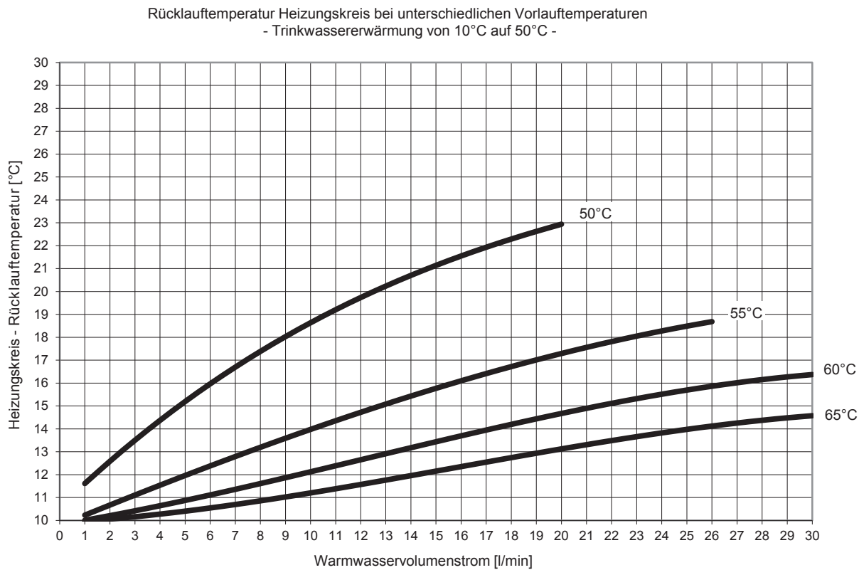
Abb. 70: Leistungsbereich 3, Trinkwassererwärmung auf 50 °C
