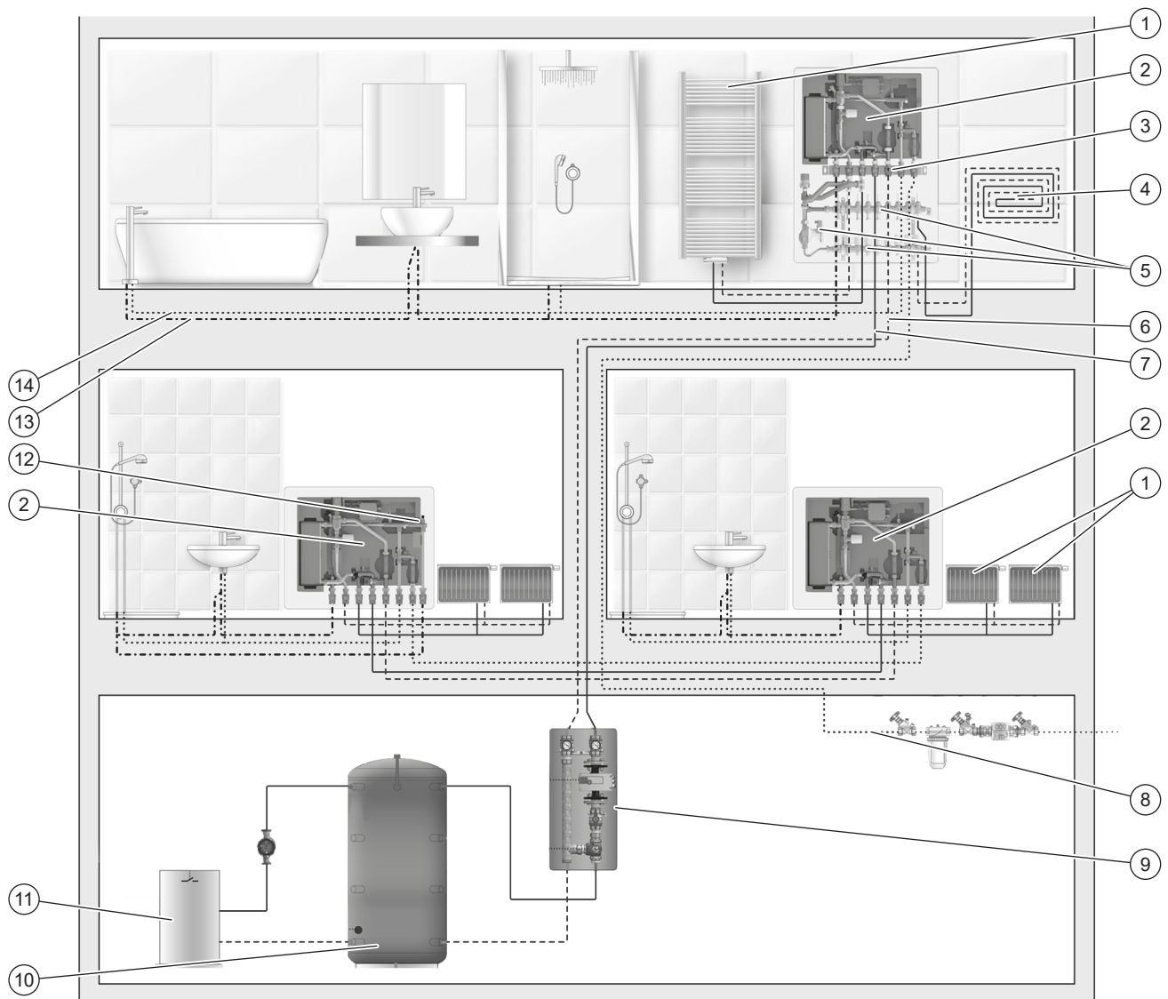
Abb. 8: Anlagenschema: Wohnungsstation
