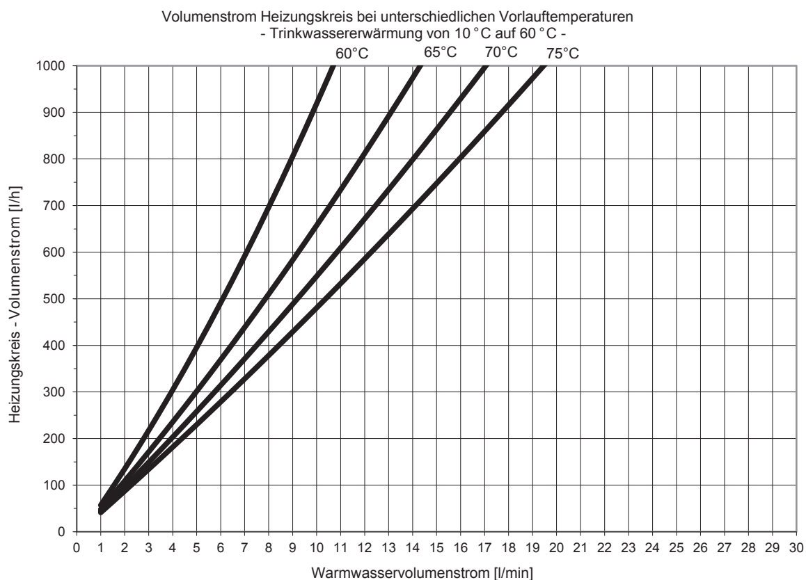
Abb. 57: Leistungsbereich 1, Trinkwassererwärmung auf 60 °C
