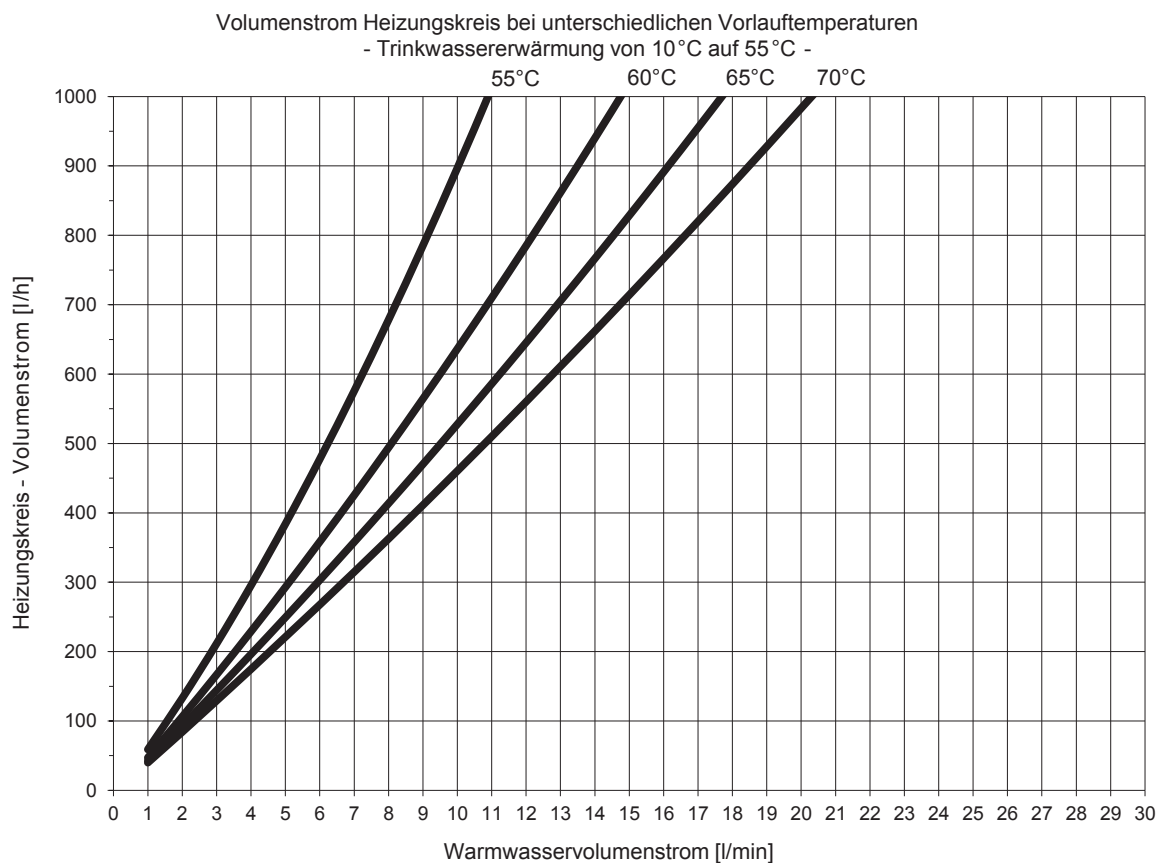
Abb. 55: Leistungsbereich 1, Trinkwassererwärmung auf 55 °C
