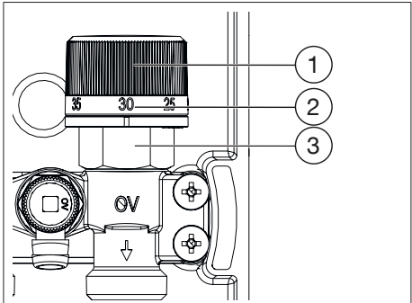
Fig. 4 : Poignée manuelle
