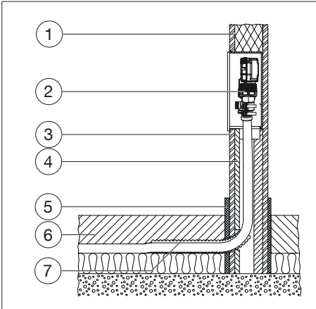
Abb. 7: Einbauquerschnitt
