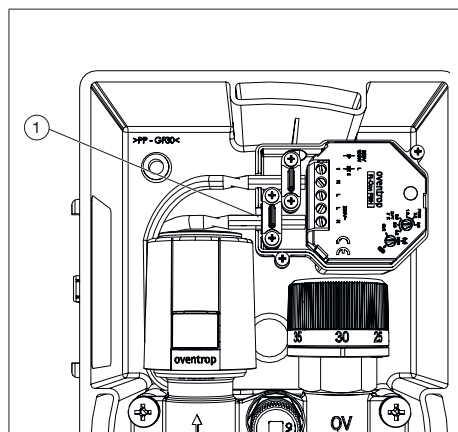
Fig. 10 : Branchement électrique du récepteur radio « R-Con FBH »
