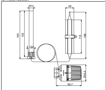
Dimensiuni
