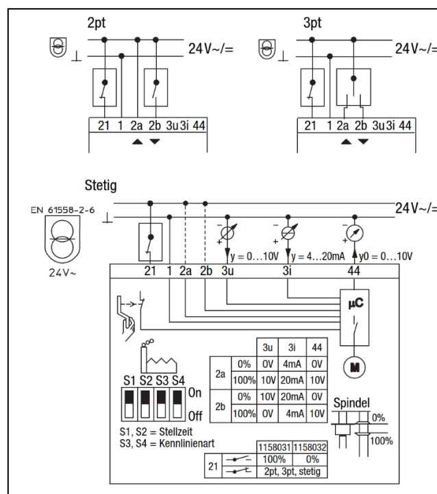
Schaltpläne, Art.-Nr. 1158031/32
