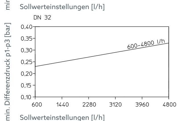
Abb. 13: Mindest-Differenzdrücke
