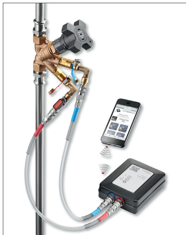
Messsystem „OV-DMC 3“ Art.-Nr. 1069278 mit „Hydrocontrol VTR“
