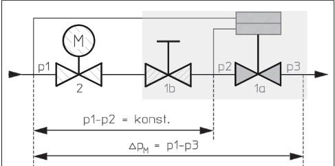
Illustr. 3: Funcionamiento de la “Cocon QTZ”, PN 25
