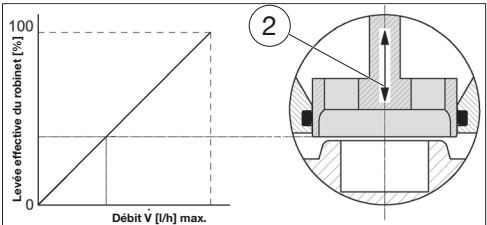
Fig. 5: Courbe de fonctionnement de l'unité de régulation
