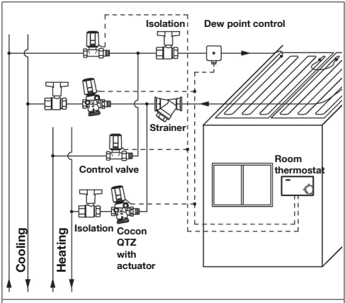
Illustr. 7: Ejemplo de instalación 2: Sistema de 4 tubos
