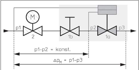
Fig. 3: Principe du fonctionnement «Cocon QTZ», PN 25
