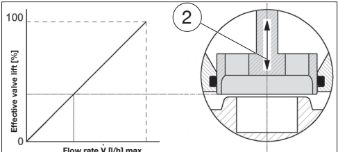
Illustr. 5: Curva característica lineal de la unidad de regulación
