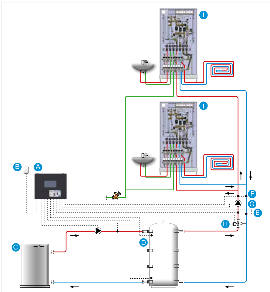
Systeem opbouw
