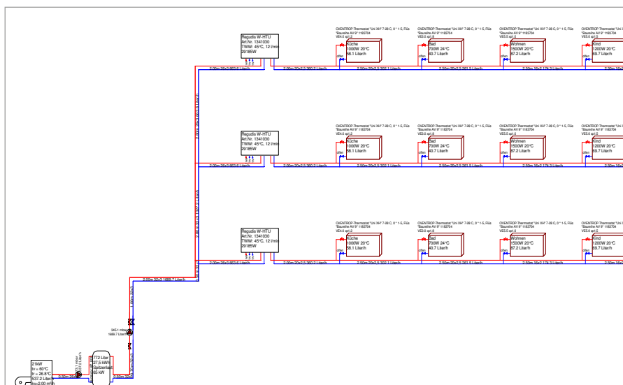
Een andere mogelijk is de radiatoren voorbij het woningstation in te tekenen en er een vermogen aan toe te kennen. OVplan telt de vermogens van de radiatoren dan op.
