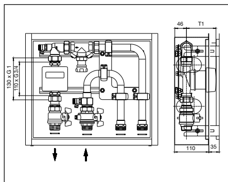
Abb. 5.1: Einbautiefe „Floorbox“
