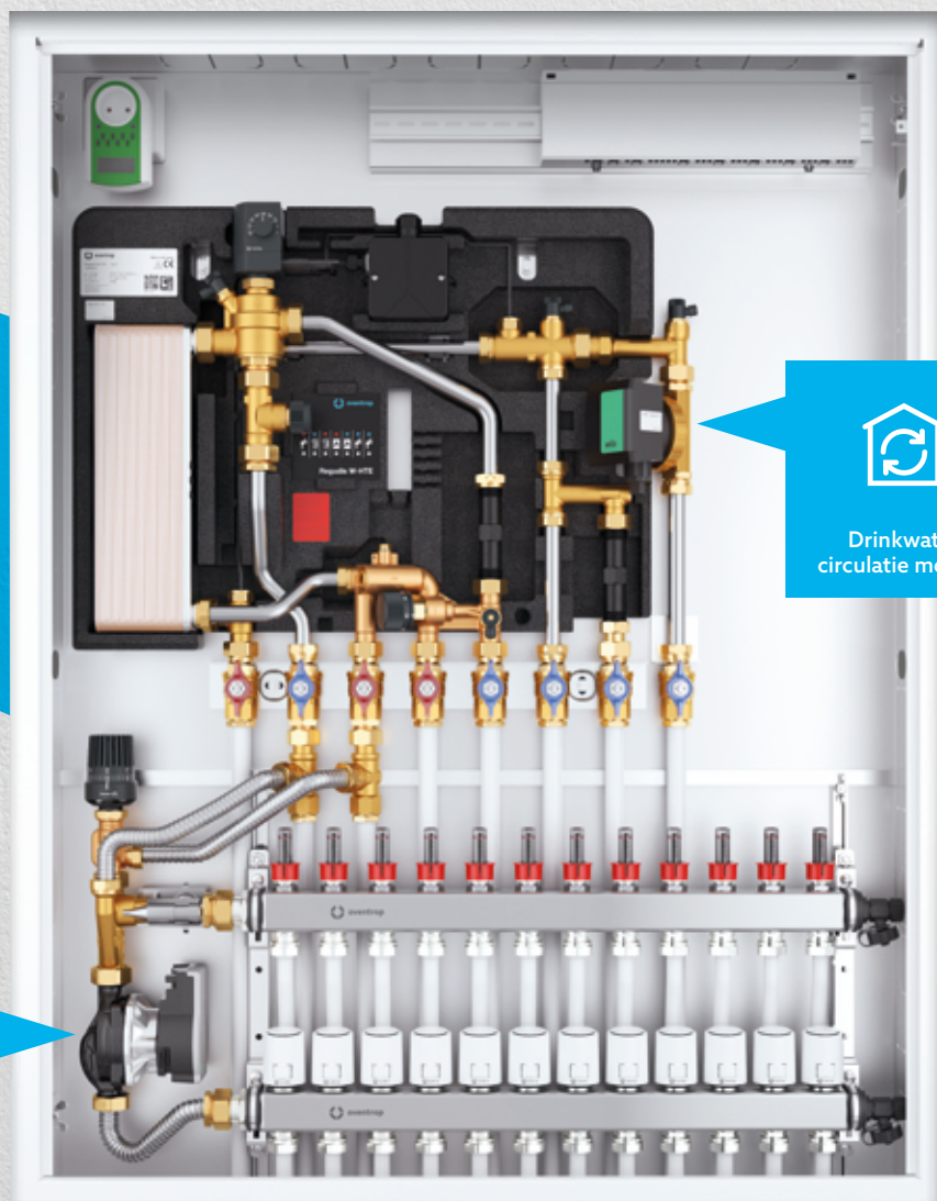
Aanvoertemperatuur regelmodule
