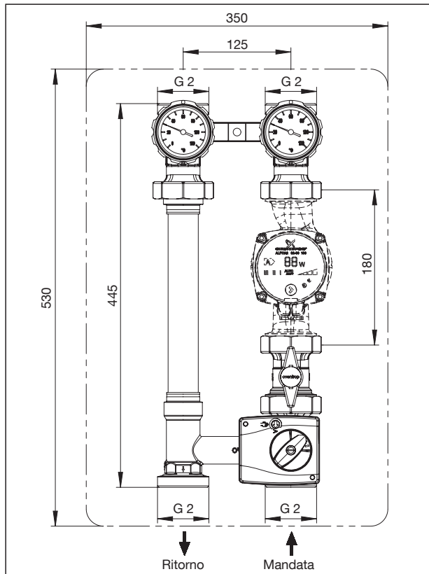
Dimensioni "Regumat M3-180" DN 32
