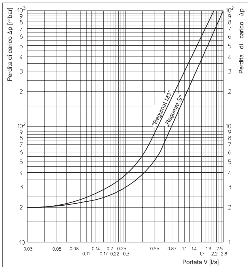
Diagramma delle portate
