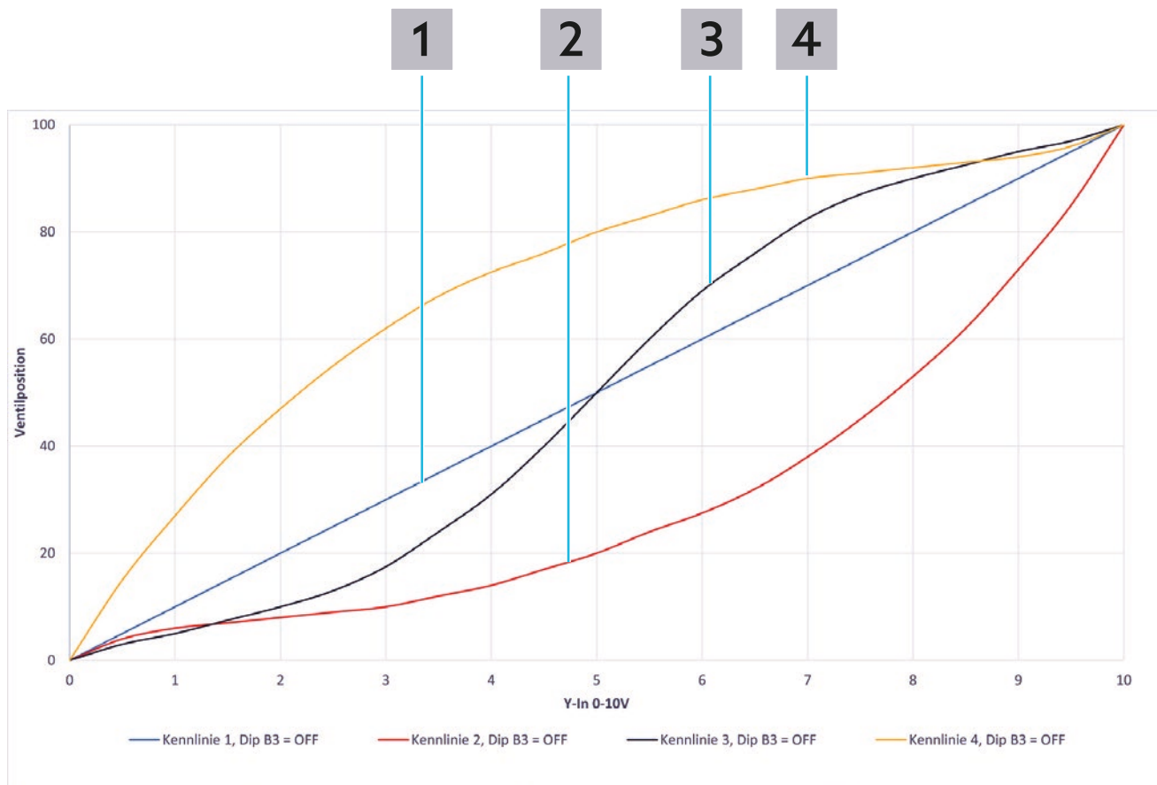
Abb. 28: Kennlinien
