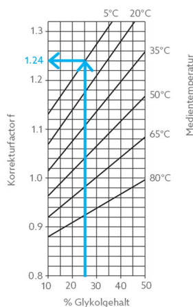
Korrekturfaktor f für Propylen Glykol
