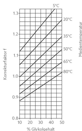
Korrekturfaktor f für Ethylen Glykol
