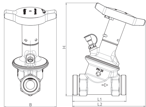
Fig. 3: Encombrements vue de côté / vue de face - Version avec filetage mâle
