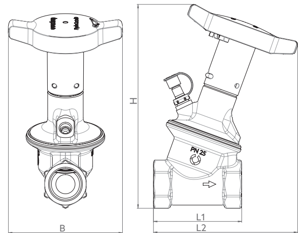
Fig. 2: Encombrements vue de côté / vue de face - Version avec filetage femelle
