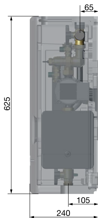
Fig. 7: Encombrements Regumaq X-25 vue de côté
