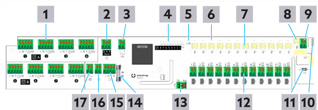
Abb. 5: Platine mit Klemmen und Statusanzeigen
