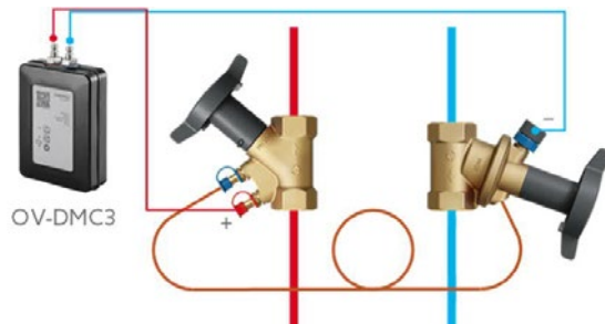
Abb. 7: Anschlusschema OV-DMC3
