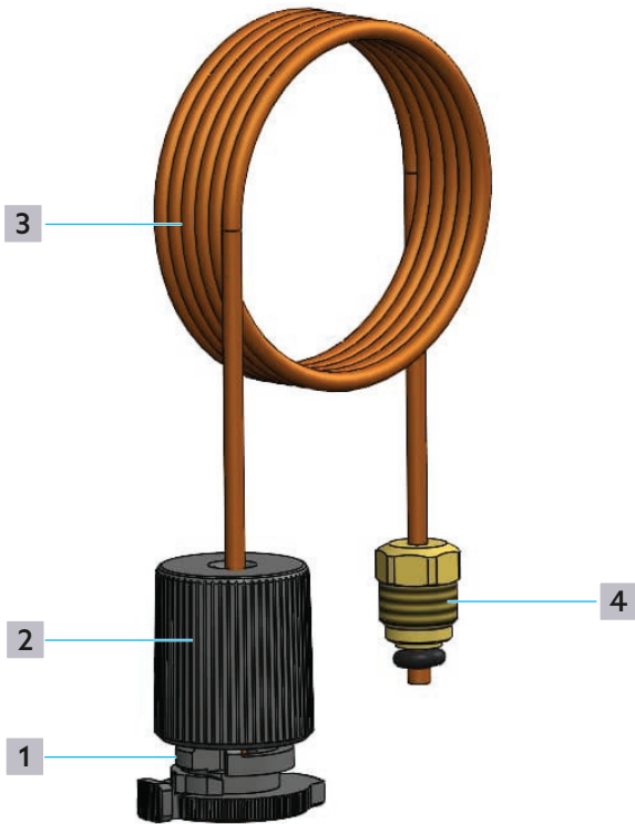
图 4： 安装脉冲管道
