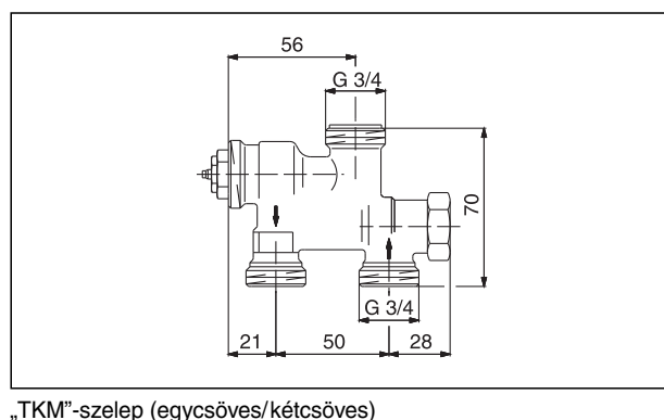
„TKM”-szelep (egycsöves/kétcsöves)
