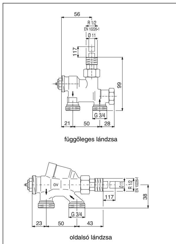
Lánczásszelep (egycsöves/kétcsöves)
