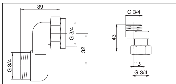
S-csatlakozócsavarzat méretei
