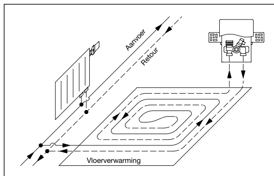
Inbouwschema „Unibox vario”, basisuitrusting
