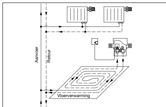
Inbouwschema „Unibox vario”, met ruimtethermostaat en stelaandrijving
