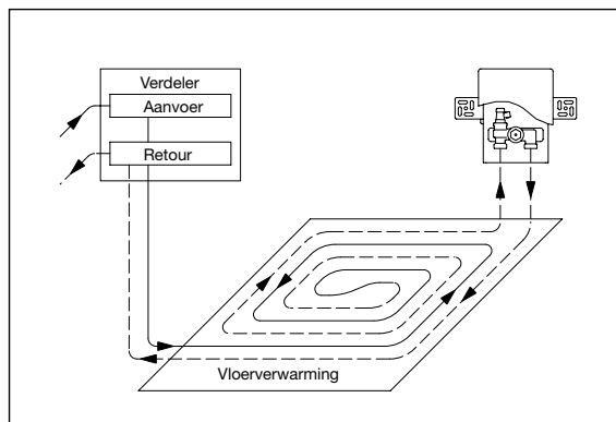
Inbouwschema temperatuurregeling per vertrek
