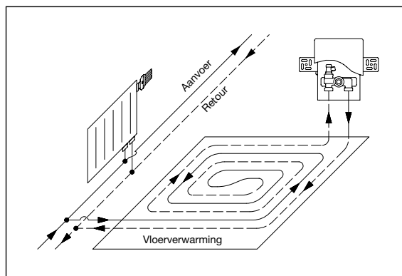
Inbouwschema retourwatertemperatuurbegrenzing
