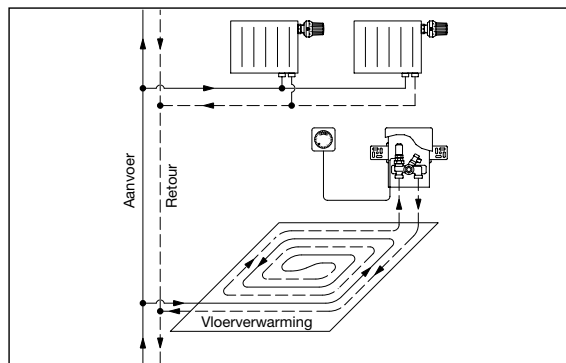
Inbouwschema „Unibox vario”, met thermostaat met afstandsbediening „Uni LH”
