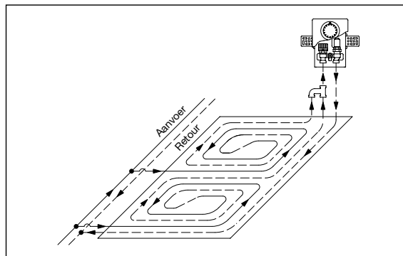
Inbouwschema „Unibox”, met twee even lange cv-circuits
