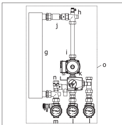
Моновалентен резервоар (вторичен кръг)
