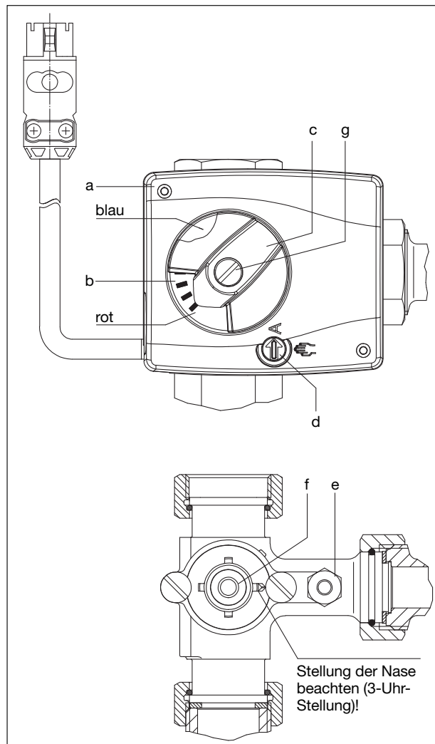
Montage Stellmotor
