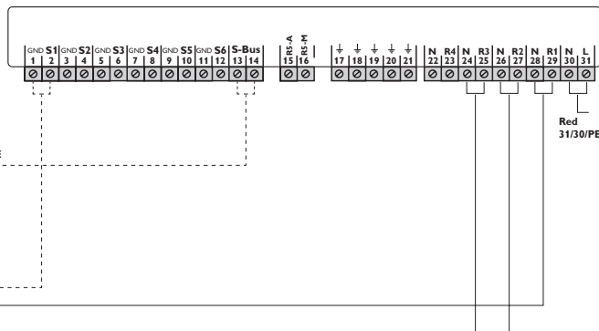
Módulo Regtronic EM 1 como circuito de calentamiento con mezcla 2
