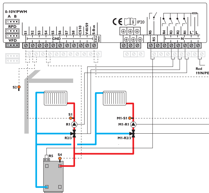
Módulo Regtronic EM 1 como circuito de calentamiento con mezcla 2
