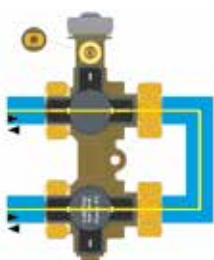
Normaal bedrijf
