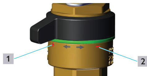
Fig. 3: Position de la poignée ouverte / fermée
