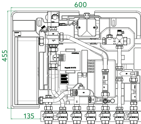
Fig. 7: Dimensions de la station d'appartement Regudis W-HTE en mm
